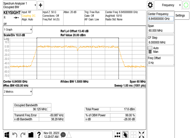
802.11n_40MHz_Chain1_6845MHz
