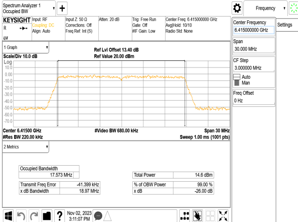
802.11n_20MHz_Chain2_6415MHz
