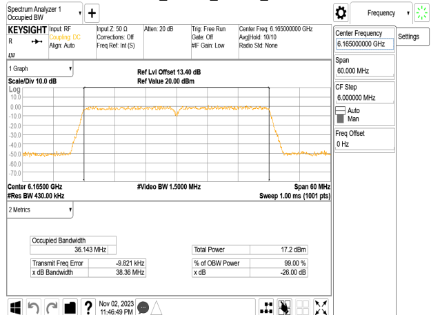
802.11n_40MHz_Chain2_6165MHz
