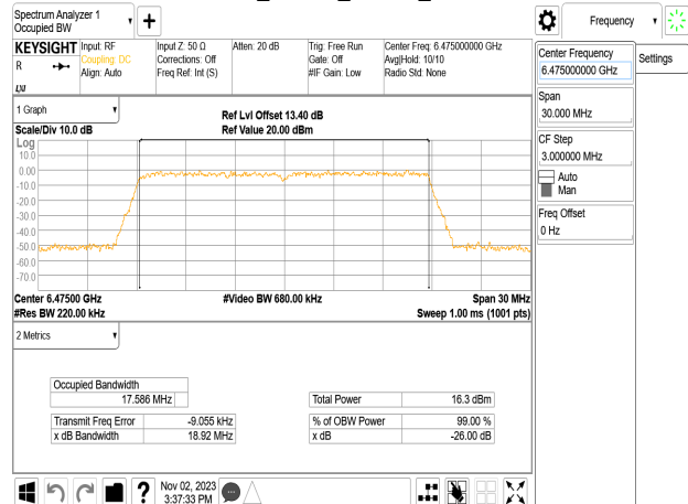
802.11n_20MHz_Chain3_6475MHz
