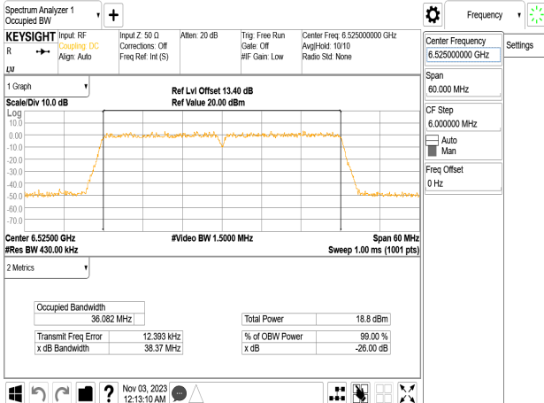
802.11n_40MHz_Chain1_6525MHz
