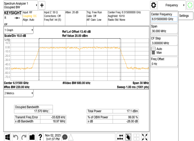
802.11n_20MHz_Chain2_6515MHz
