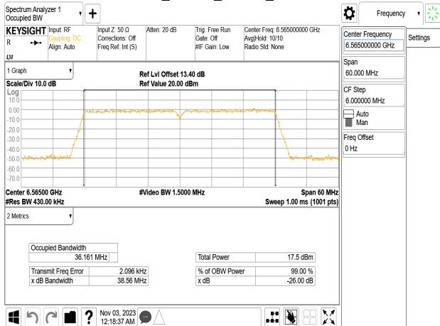
802.11n_40MHz_Chain0_6565MHz
