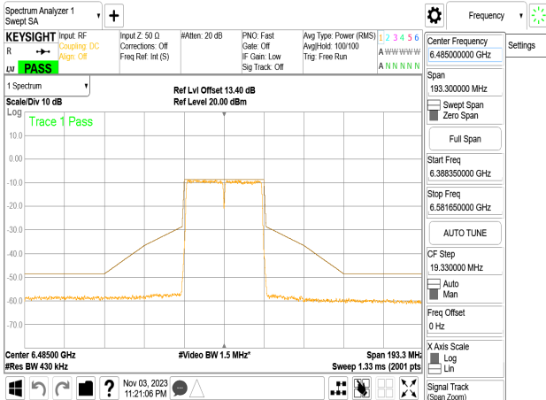
802.11n_40MHz_Chain0_6485MHz
