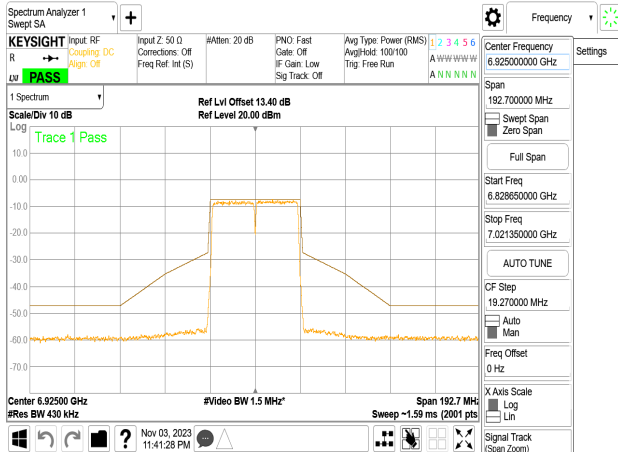
802.11n_40MHz_Chain0_6925MHz
