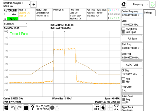
802.11n_40MHz_Chain1_6565MHz
