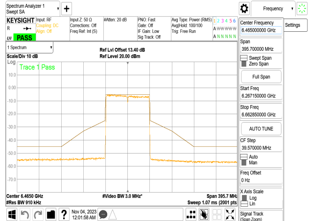
802.11ac_80MHz_Chain0_6465MHz
