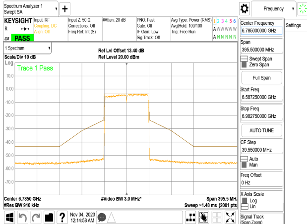
802.11ac_80MHz_Chain1_6785MHz
