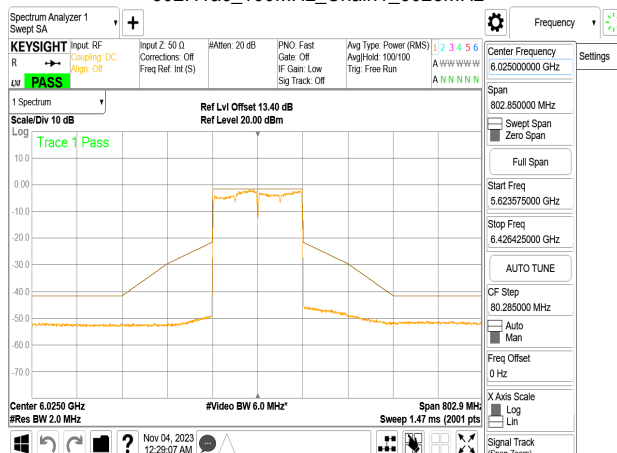
802.11ac_160MHz_Chain1_6025MHz
