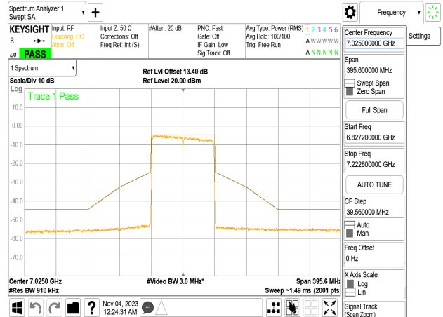
802.11ac_80MHz_Chain1_7025MHz
