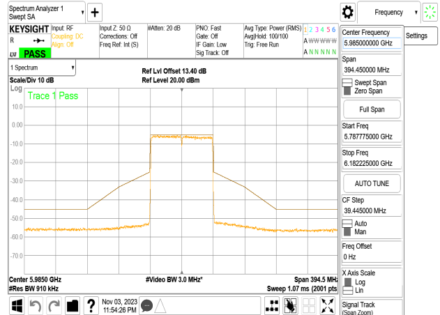
802.11ac_80MHz_Chain3_5985MHz
