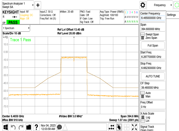
802.11ac_80MHz_Chain3_6465MHz
