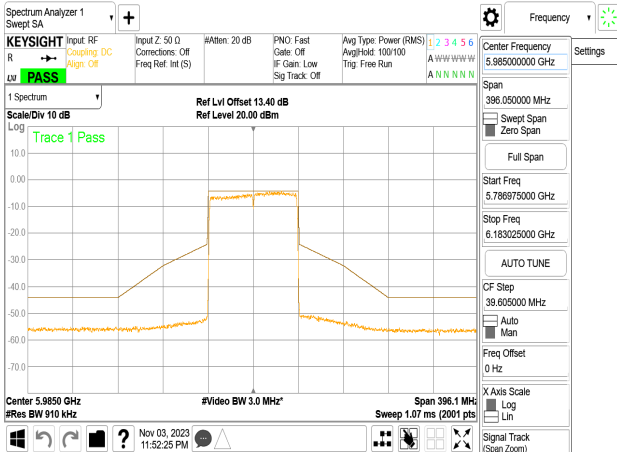
802.11ac_80MHz_Chain0_5985MHz
