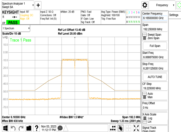
802.11n_40MHz_Chain3_6165MHz
