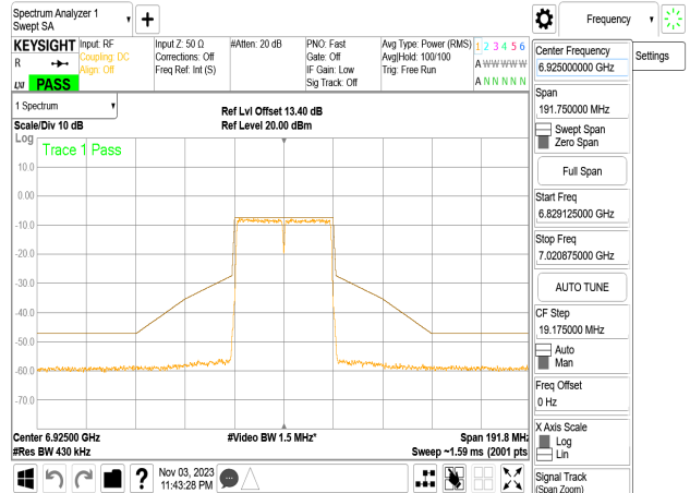
802.11n_40MHz_Chain3_6925MHz
