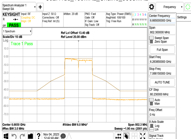
802.11ac_160MHz_Chain0_6665MHz
