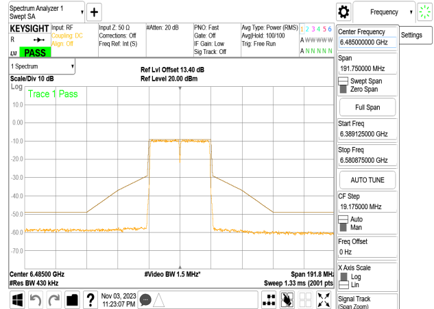
802.11n_40MHz_Chain3_6485MHz
