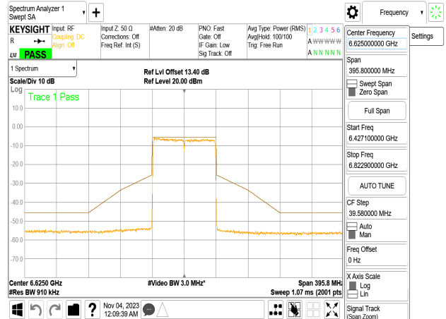
802.11ac_80MHz_Chain2_6625MHz
