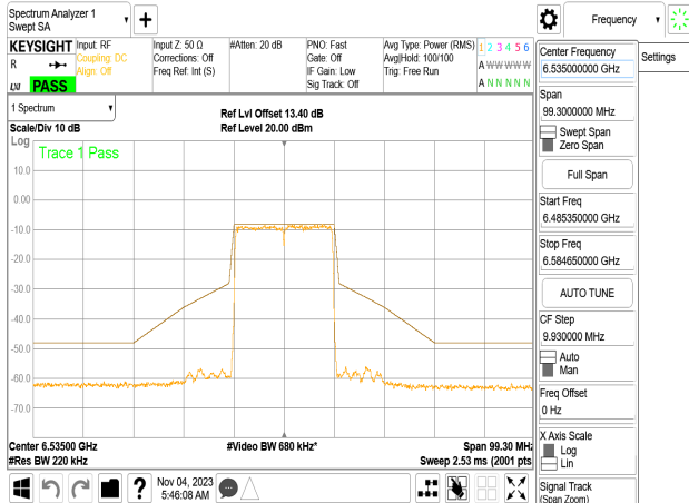
802.11be_20MHz_Chain0_6535MHz
