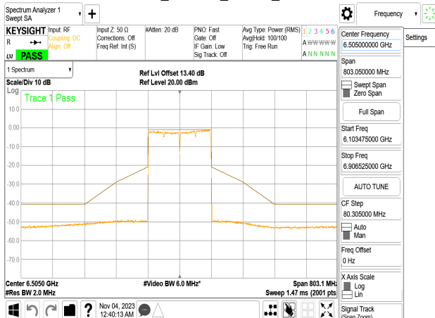
802.11ac_160MHz_Chain1_6505MHz
