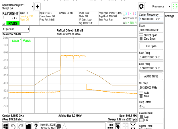
802.11ac_160MHz_Chain3_6185MHz
