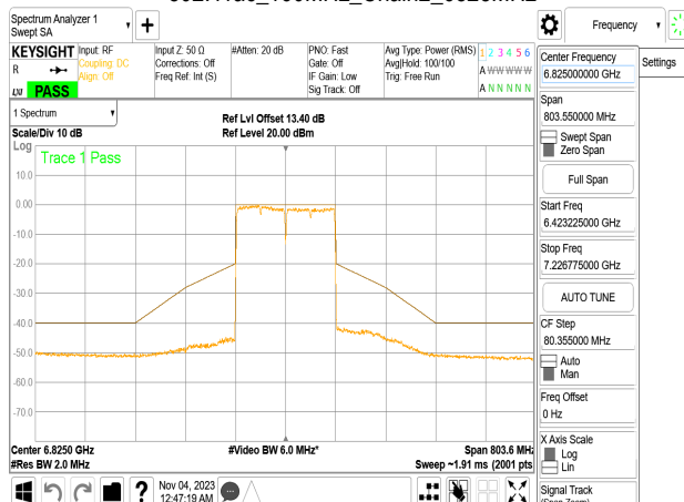
802.11ac_160MHz_Chain2_6825MHz
