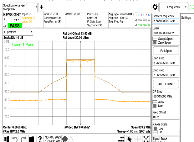
802.11ac_160MHz_Chain3_6665MHz
