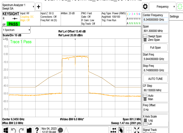
802.11ac_160MHz_Chain2_6345MHz
