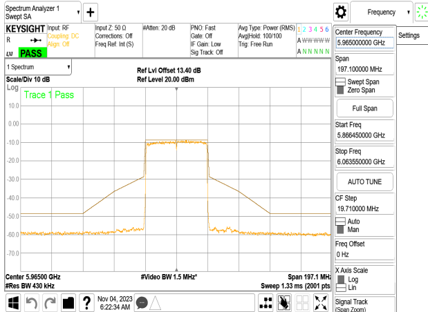
802.11be_40MHz_Chain2_5965MHz
