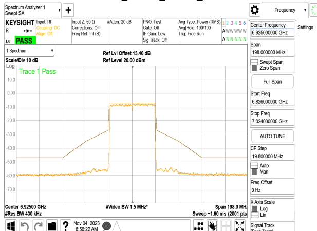
802.11be_40MHz_Chain1_6925MHz
