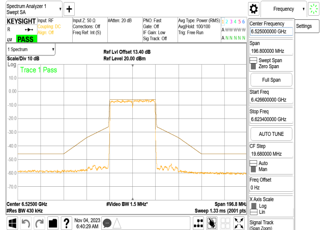
802.11be_40MHz_Chain0_6525MHz
