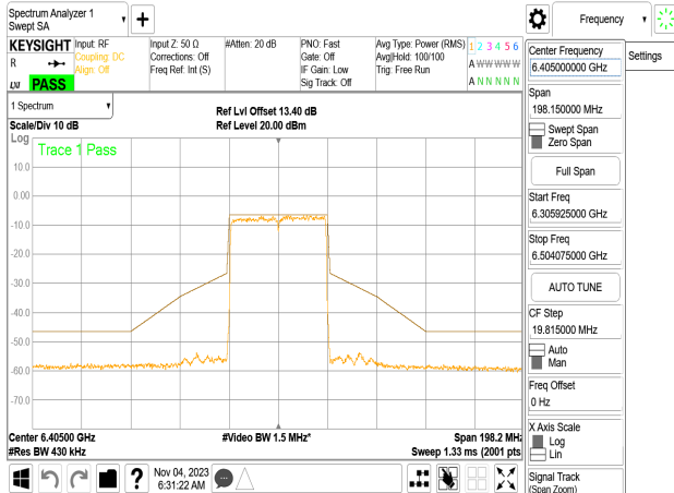
802.11be_40MHz_Chain0_6405MHz
