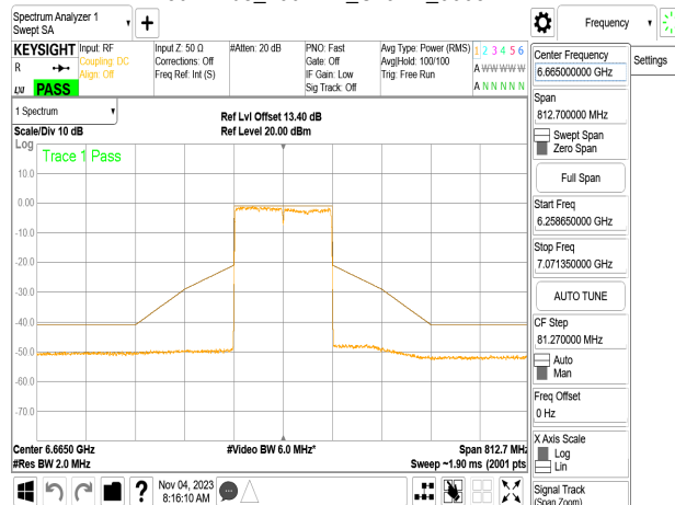
802.11be_160MHz_Chain1_6665MHz
