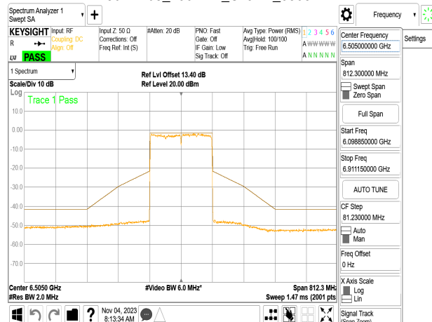
802.11be_160MHz_Chain2_6505MHz
