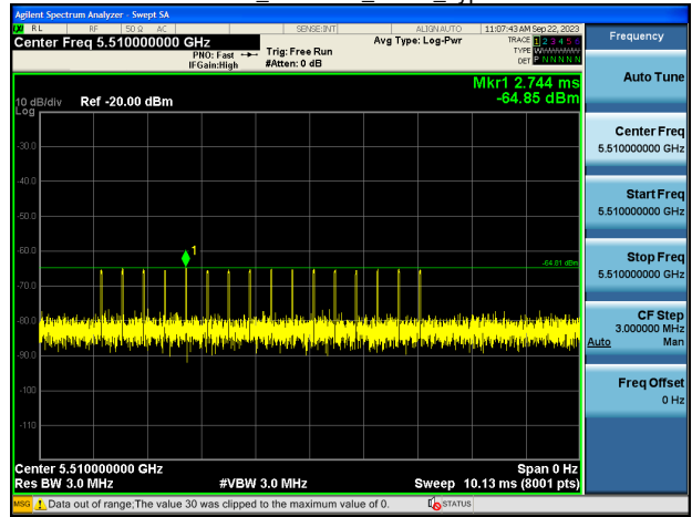
EHT40_5510MHz_Radar_Type 5
