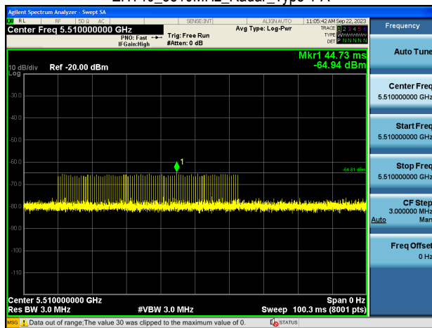
EHT40_5510MHz_Radar_Type 1-A
