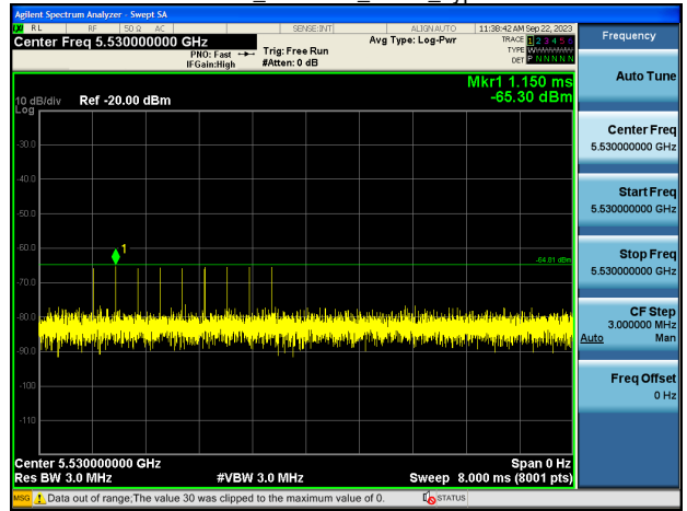
EHT80_5530MHz_Radar_Type 6
