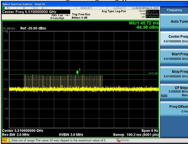
EHT40_5510MHz_Radar_Type 2
