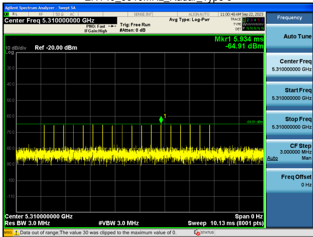
EHT40_5310MHz_Radar_Type 4
