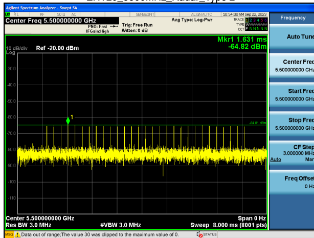
EHT20_5500MHz_Radar_Type 3
