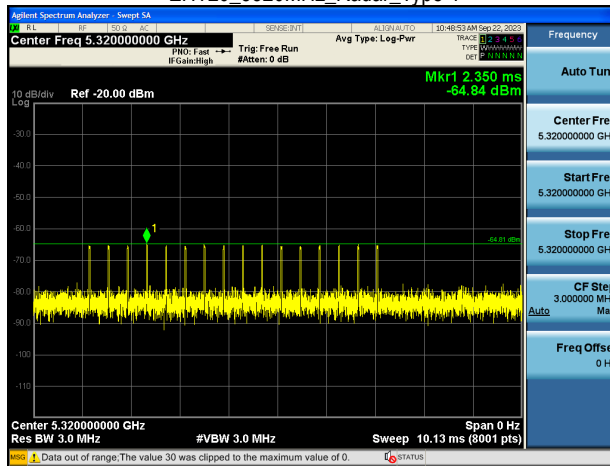
EHT20_5320MHz_Radar_Type 5
