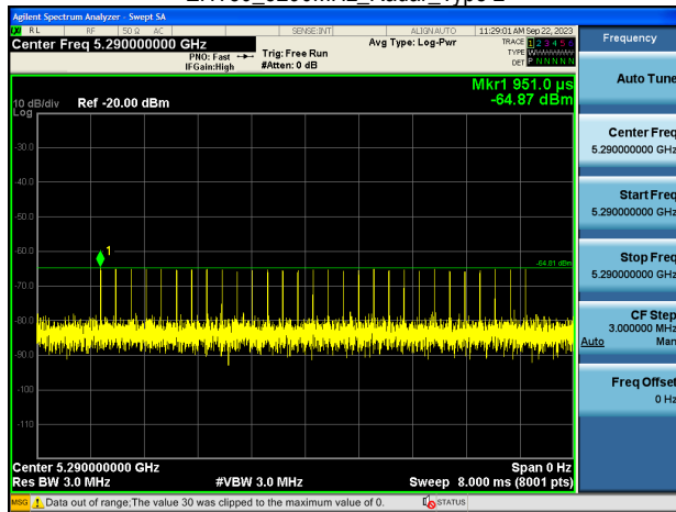
EHT80_5290MHz_Radar_Type 3
