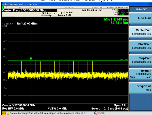
EHT20_5320MHz_Radar_Type 3
