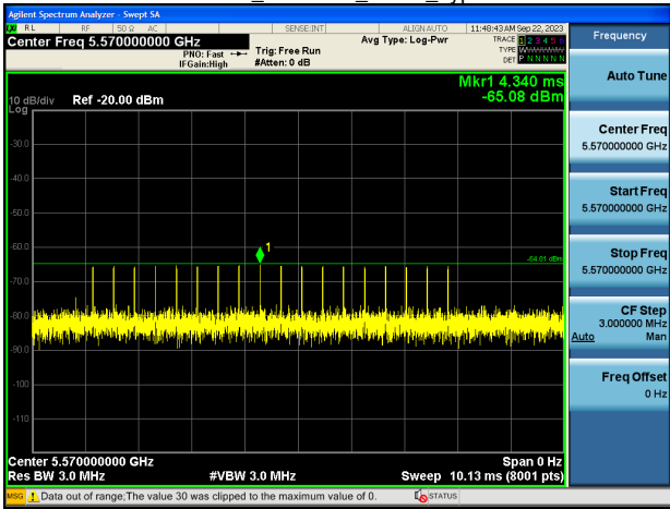
EHT160_5570MHz_Radar_Type 4
