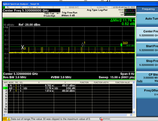
EHT20_5320MHz_Radar_Type 6
