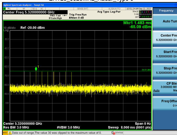
EHT20_5320MHz_Radar_Type 6
