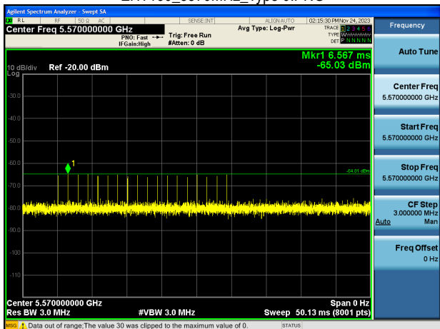
EHT160_5570MHz_Type 0.PNG
