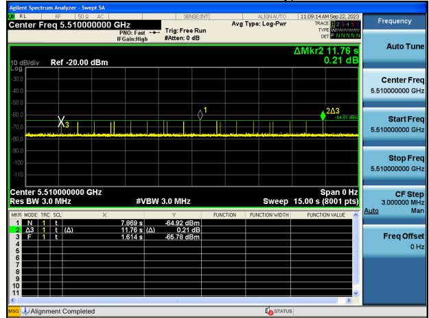
EHT40_5510MHz_Radar_Type 6
