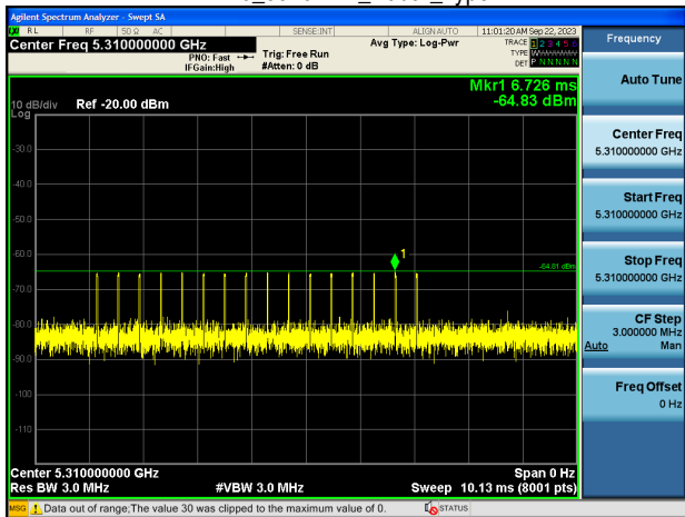
EHT40_5310MHz_Radar_Type 5
