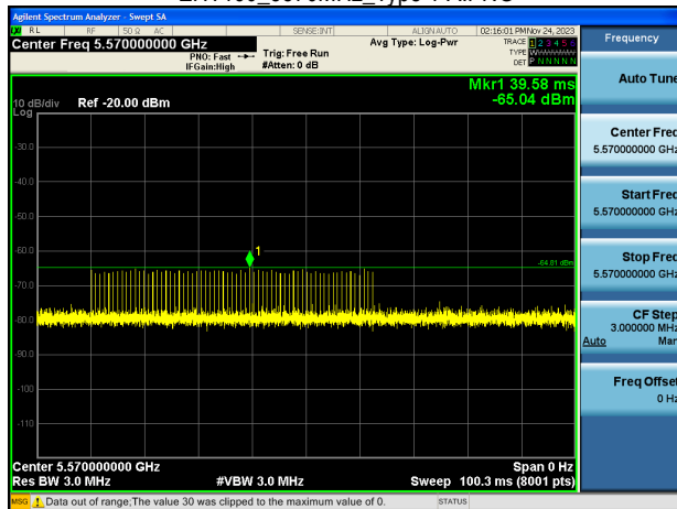
EHT160_5570MHz_Type 1-B.PNG
