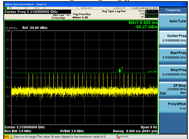
EHT40_5310MHz_Radar_Type 2
