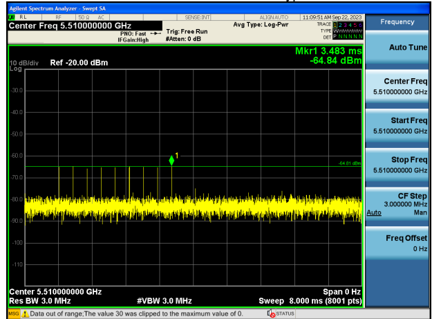
EHT40_5510MHz_Radar_Type 6
