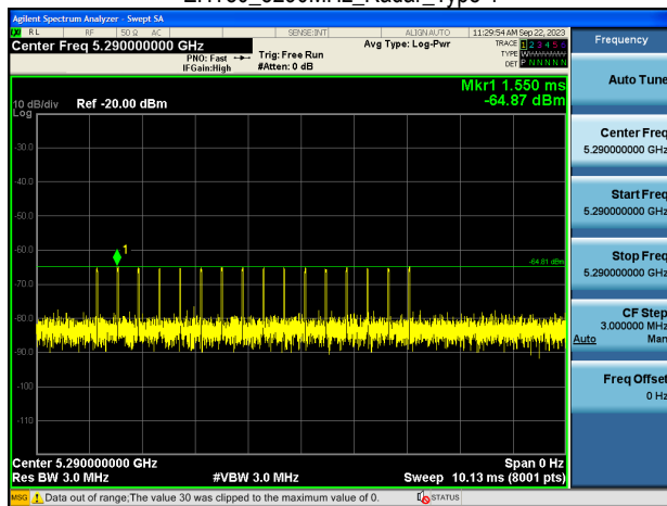
EHT80_5290MHz_Radar_Type 4
