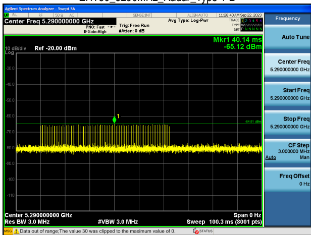
EHT80_5290MHz_Radar_Type 1-B
