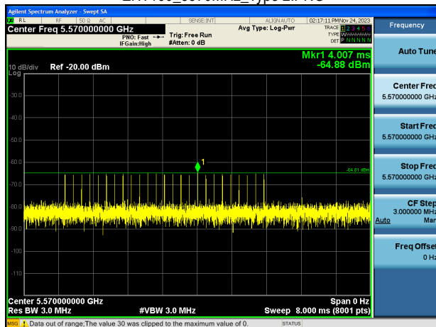
EHT160_5570MHz_Type 2.PNG
