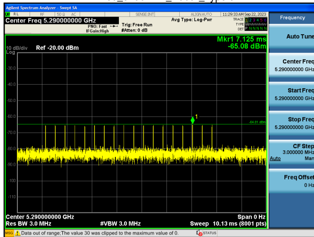
EHT80_5290MHz_Radar_Type 4
