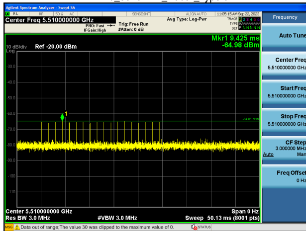
EHT40_5510MHz_Radar_Type 1-A
