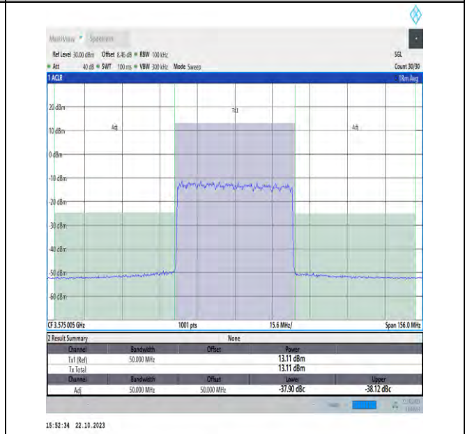
NTNV_N48_PC3_30_50_L_TID16_#1_-50_50
