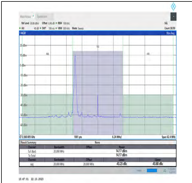
NTVN_N48_PC3_30_20_L_TID18_#1_-15_15
