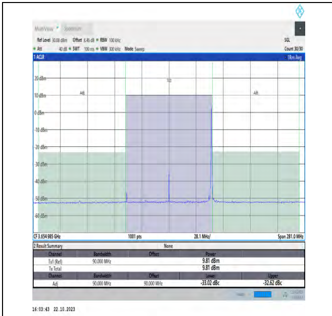
NTV_N48_PC3_30_90_H_TID18_#1_90_90
