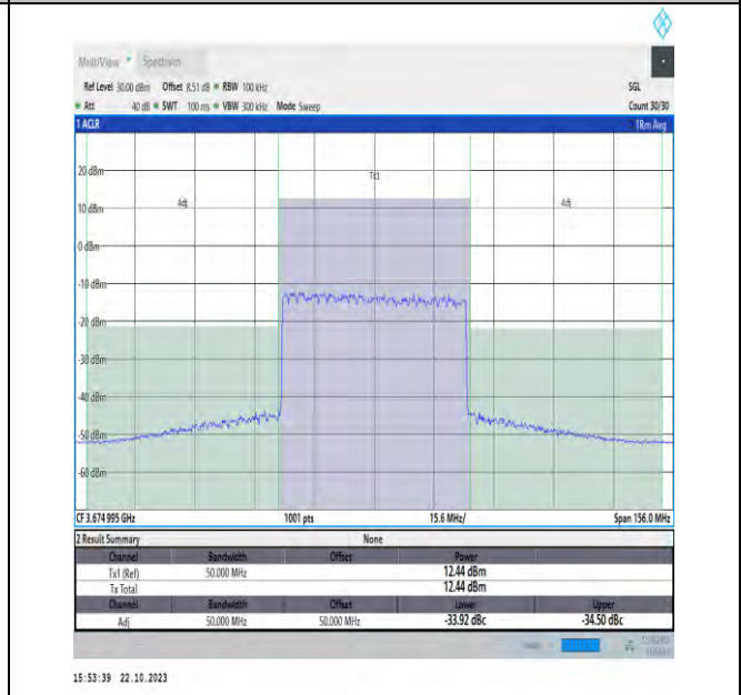
NTVN_N48_PC3_30_50_H_TID16_#1_-50_50
