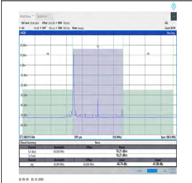
NTVN_N48_PC3_30_60_L_TID2_#1_-60_60
