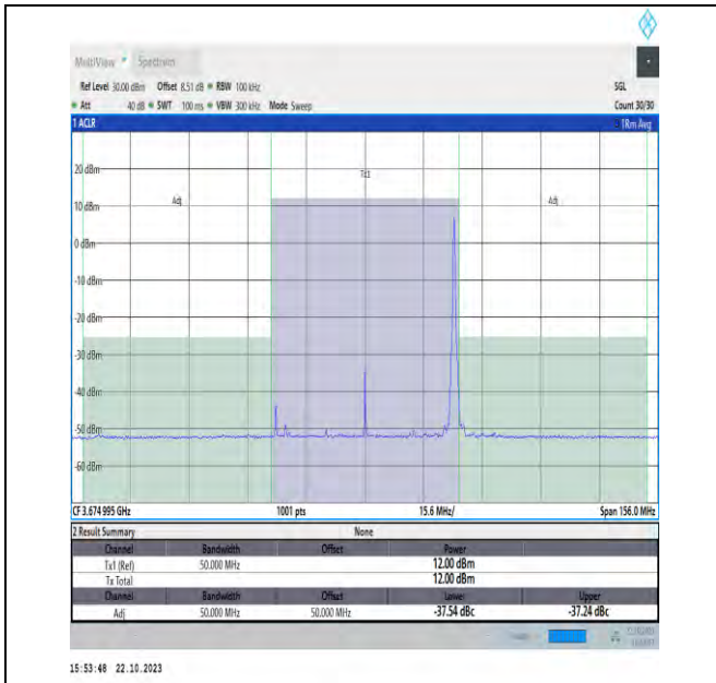
NTVN_N48_PC3_30_50_H_TID18_#1_-50_50
