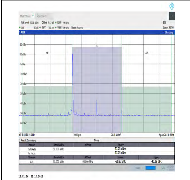
NTVN_N48_PC3_30_90_L_TID2_#1_90_90
