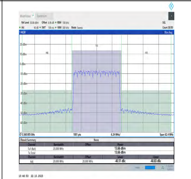
NTVN_N48_PC3_30_20_L_TID16_#1_-20_20
