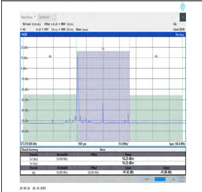
NTNV_N48_PC3_30_50_L_TID2_#1_-50_50
