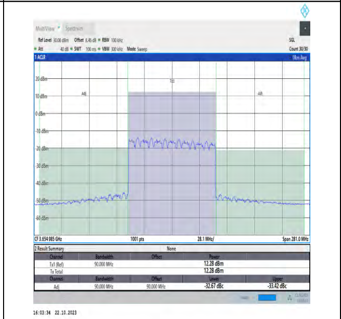
NTV_N48_PC3_30_90_H_TID16_#1_90_90
