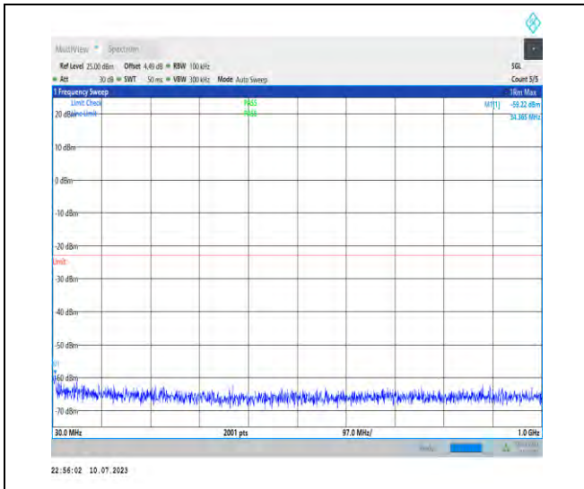
1-N66-PC3-15-40-M-1-DFT-PI2BPSK-Inner_1RB_L eft-1@1-30-1000-Ant3-34.37--59.22--23-PASS
