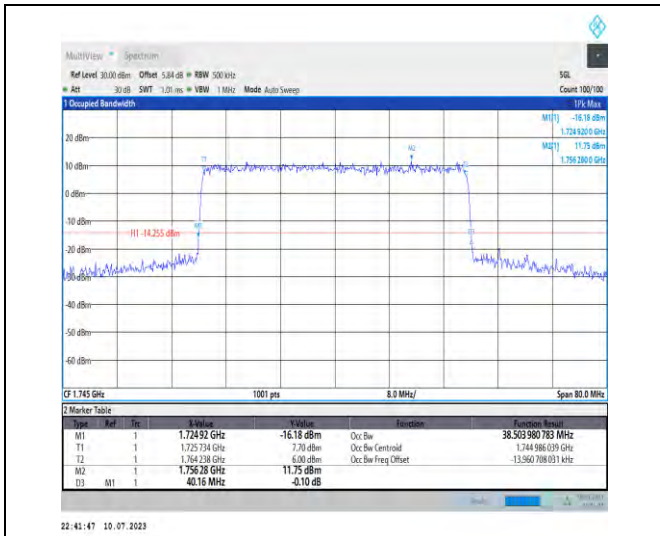
1-N66-PC3-15-40-M-7-CP-16QAM-Outer_Full-216@ 0-Ant3-38.504-40.160-≤40-PASS
