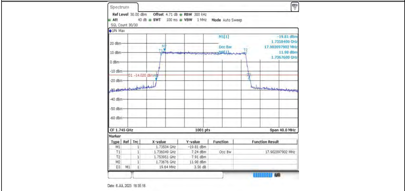
20MHz-132322 64QAM
