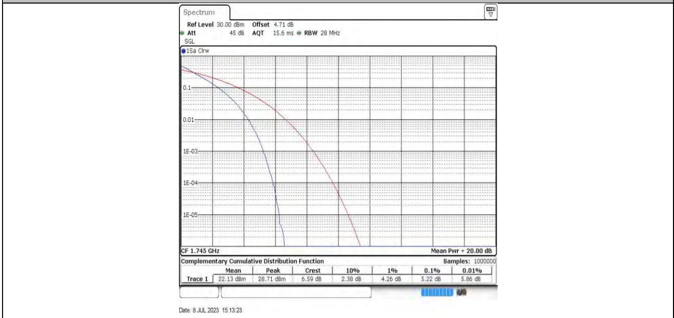
20MHz-132322 QPSK
