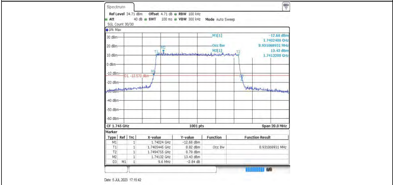
10MHz-132322 16QAM
