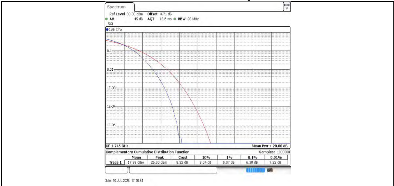
20MHz-132322 256QAM
