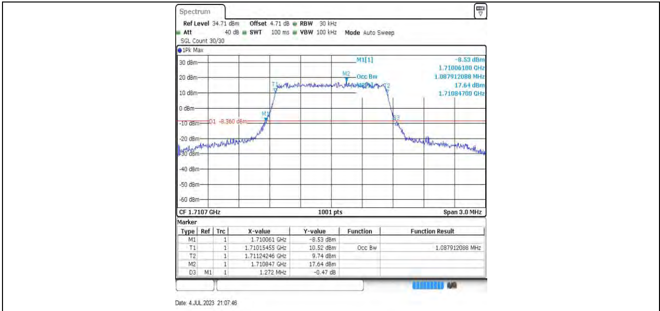
1.4MHz-131979 QPSK
