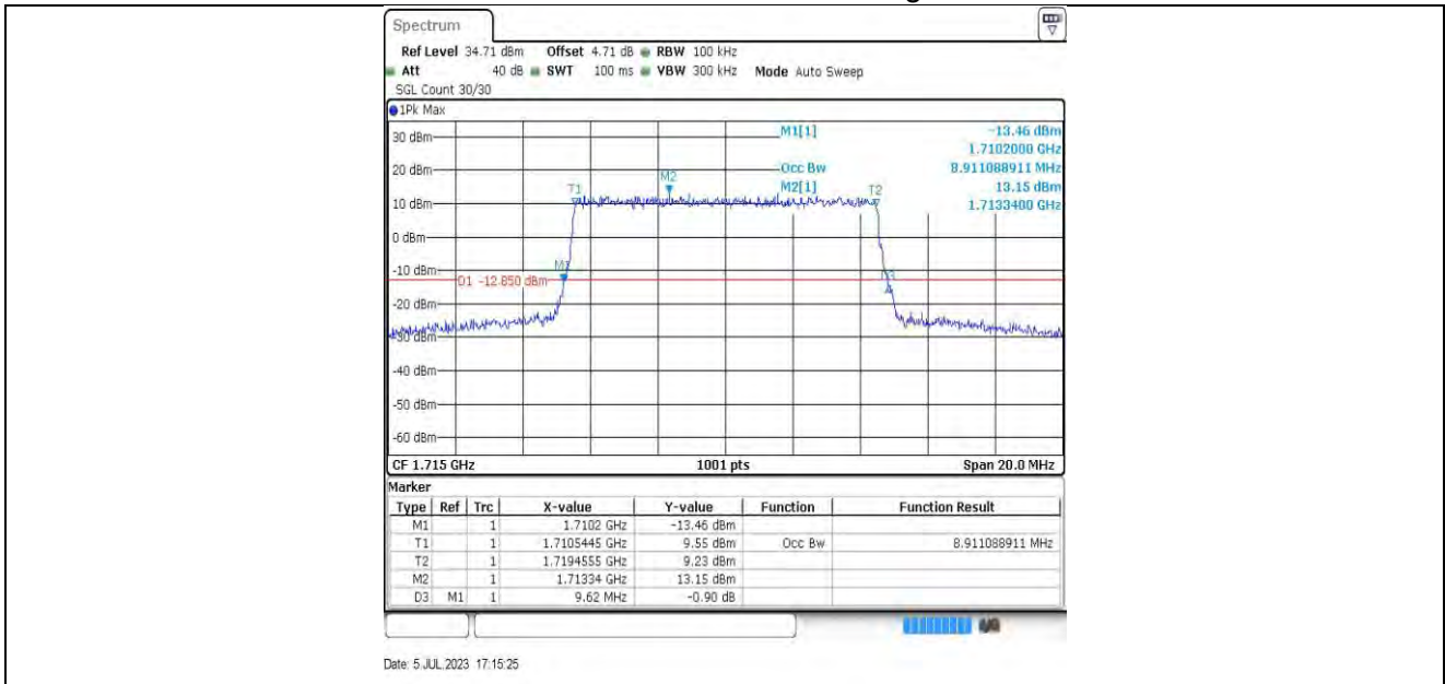
10MHz-132022 16QAM
