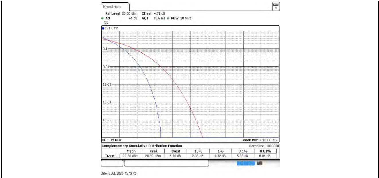
20MHz-132072 QPSK
