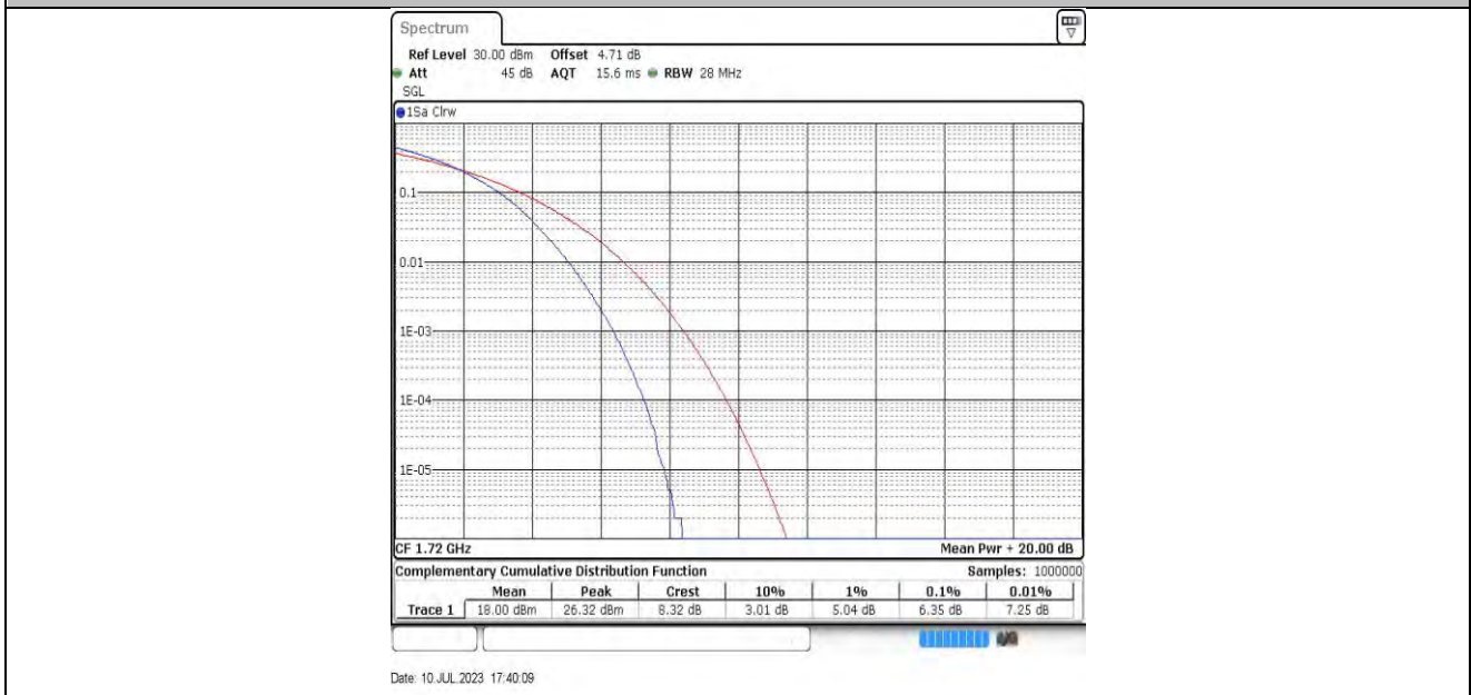
20MHz-132072 256QAM
