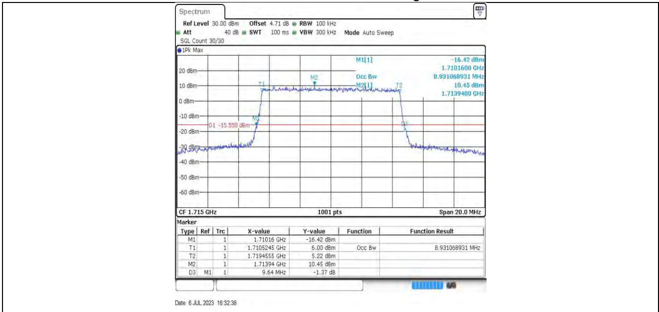
10MHz-132022 64QAM
