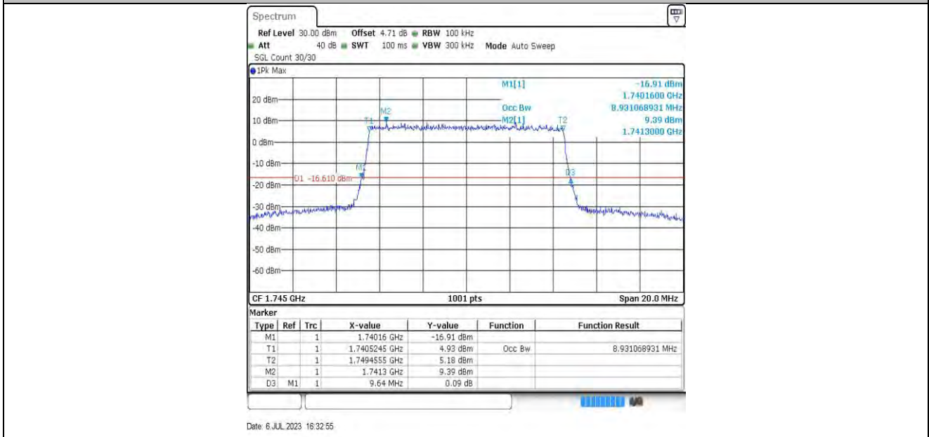
10MHz-132322 64QAM
