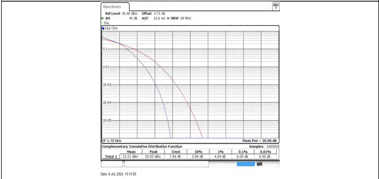
20MHz-132072 16QAM
