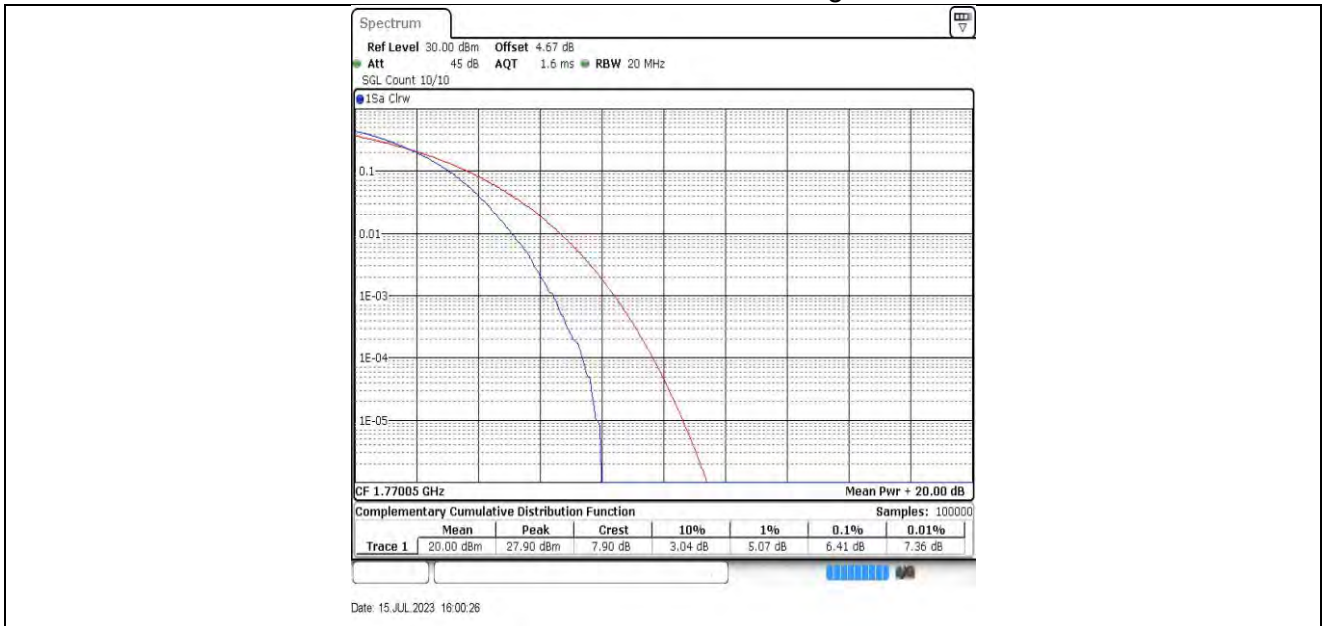
10MHz-10MHz-132523-132622 64QAM-64QAM
