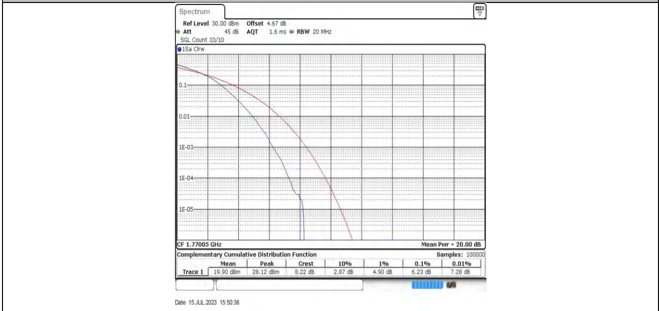
10MHz-10MHz-132523-132622 16QAM-16QAM
