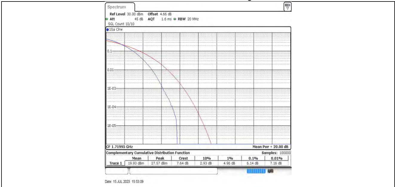
10MHz-10MHz-132022-132121 64QAM-64QAM
