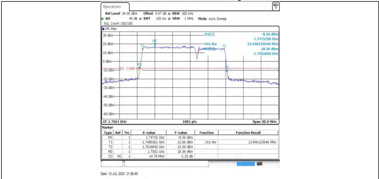
10MHz-5MHz-132397-132469 16QAM-16QAM
