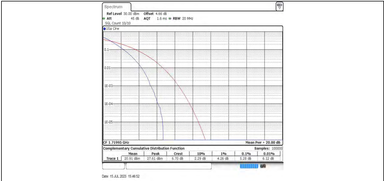
10MHz-10MHz-132022-132121 QPSK-QPSK
