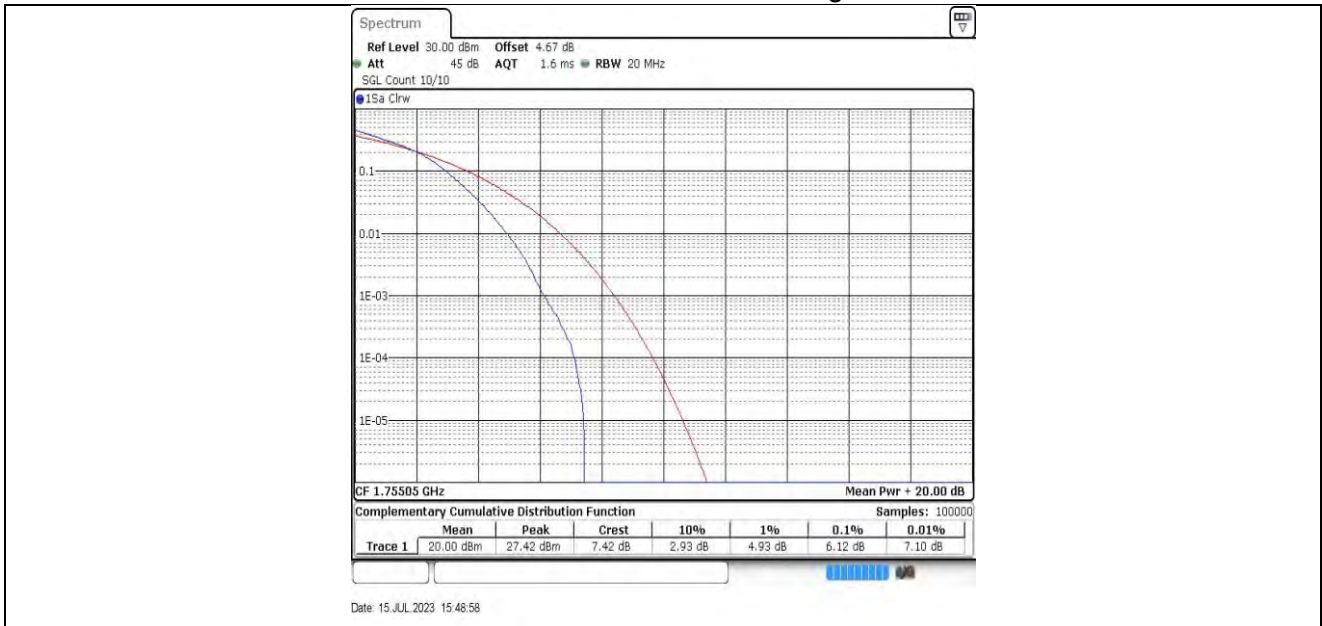
10MHz-10MHz-132373-132472 16QAM-16QAM
