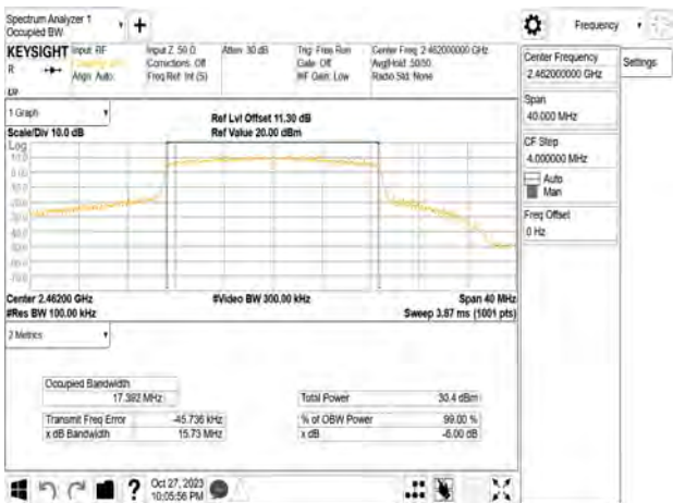
802.11n_20MHz_Chain2_2462MHz
