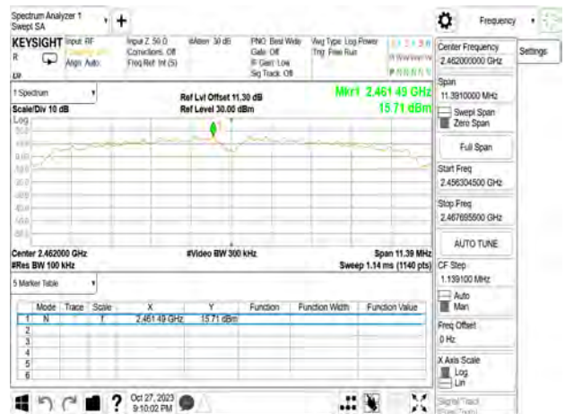
802.11b_20MHz_Chain3_2462MHz
