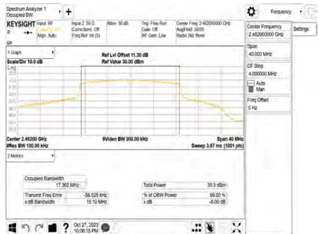
802.11n_20MHz_Chain3_2462MHz
