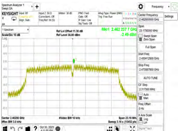
802.11g_20MHz_Chain2_2462MHz
