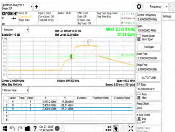
802.11be_20MHz_Chain3_2412MHz
