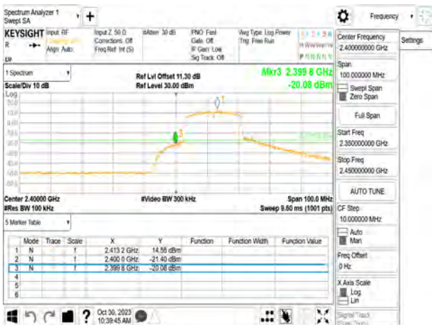
802.11n_20MHz_Chain2_2412MHz
