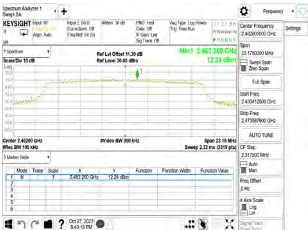
802.11g_20MHz_Chain2_2462MHz
