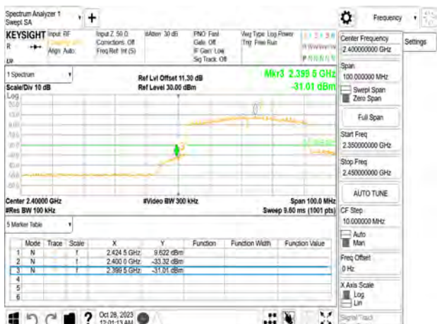
802.11be_40MHz_Chain2_2422MHz
