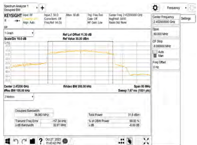
802.11be_40MHz_Chain3_2452MHz
