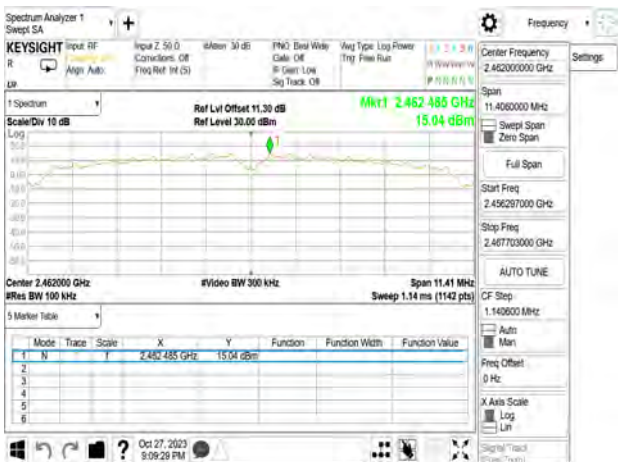
802.11b_20MHz_Chain2_2462MHz
