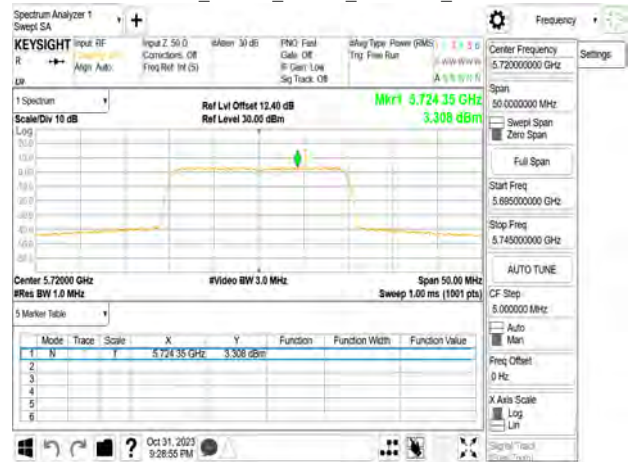
802.11be_20MHz_Chain3_5720MHz_UNII 3
