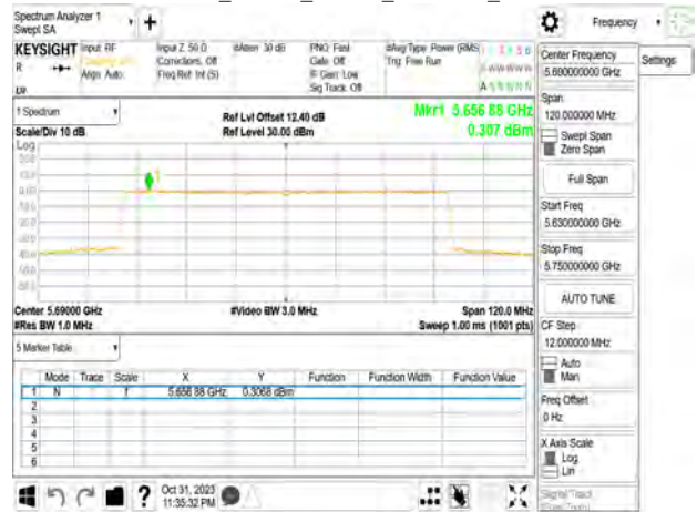
802.11be_80MHz_Chain1_5690MHz_UNII 3
