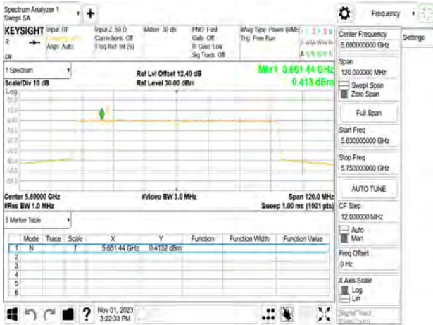
802.11ac_80MHz_Chain3_5690MHz_UNII 3
