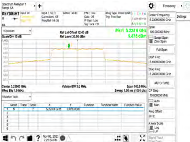
802.11n_40MHz_Chain3_5230MHz
