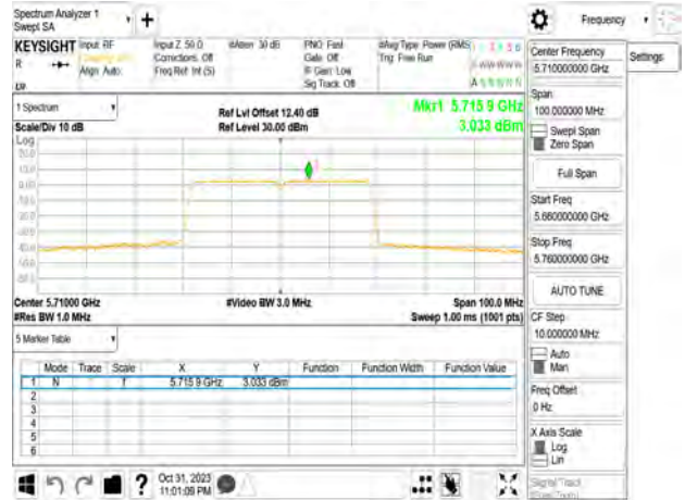
802.11n_40MHz_Chain2_5710MHz_UNII_3
