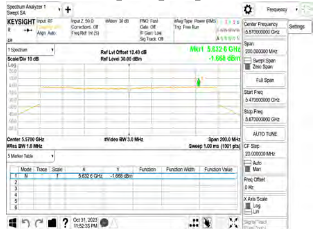
802.11be_160MHz_Chain1_5570MHz
