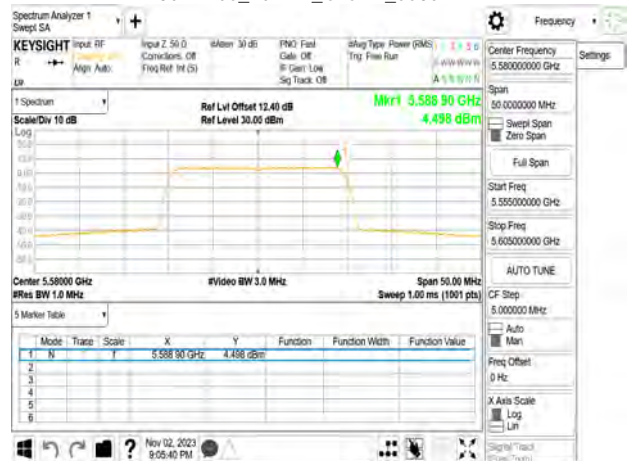
802.11be_20MHz_Chain2_5580MHz
