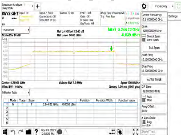
802.11ac_80MHz_Chain2_5210MHz
