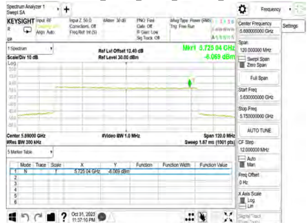
802.11be_80MHz_Chain2_5690MHz_UNII 3
