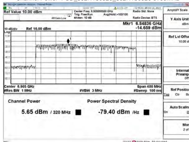
Channel Power+PSD_802.11be320_802.11be320 6905MHz
