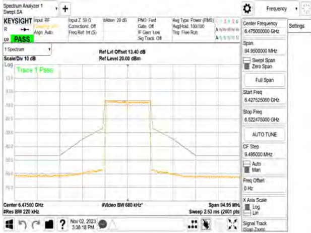
802.11n_20MHz_Chain0_6475MHz
