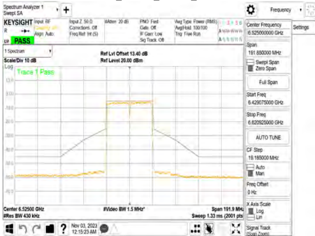
802.11n_40MHz_Chain1_6525MHz
