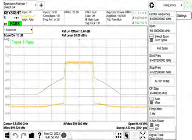
802.11n_20MHz_Chain1_6535MHz
