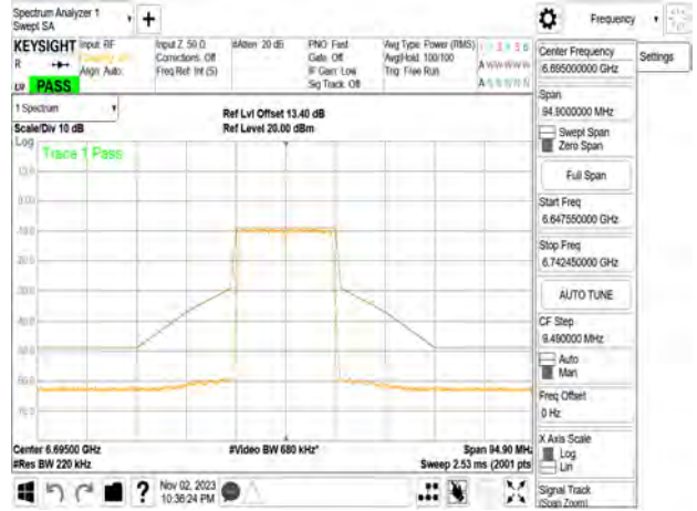
802.11n_20MHz_Chain0_6695MHz
