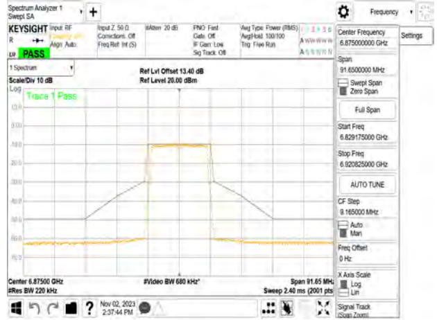
802.11a_20MHz_Chain2_6875MHz
