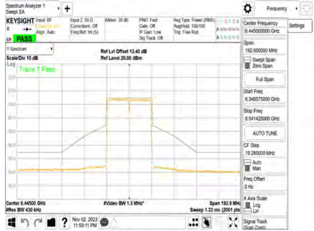
802.11n_40MHz_Chain0_6445MHz
