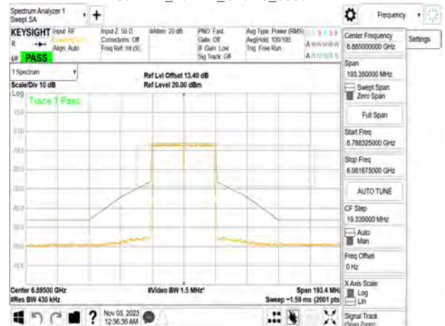
802.11n_40MHz_Chain0_6885MHz
