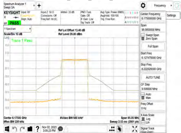
802.11n_20MHz_Chain0_6175MHz
