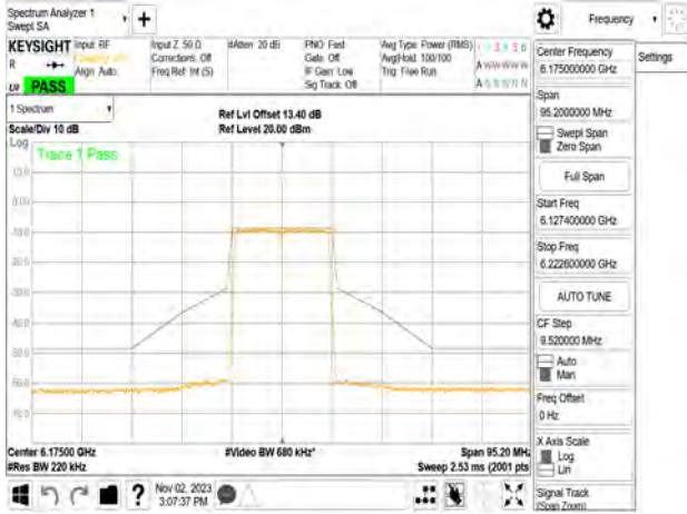
802.11n_20MHz_Chain3_6175MHz
