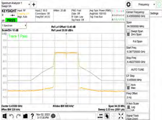
802.11n_20MHz_Chain1_6435MHz
