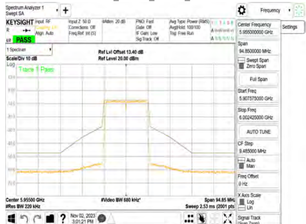
802.11n_20MHz_Chain1_5955MHz
