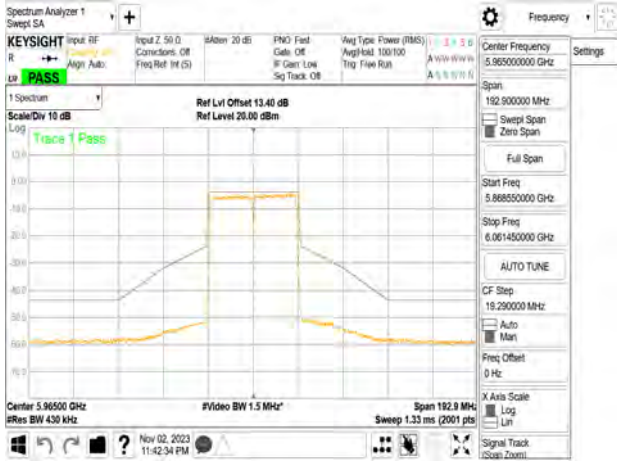
802.11n_40MHz_Chain0_5965MHz
