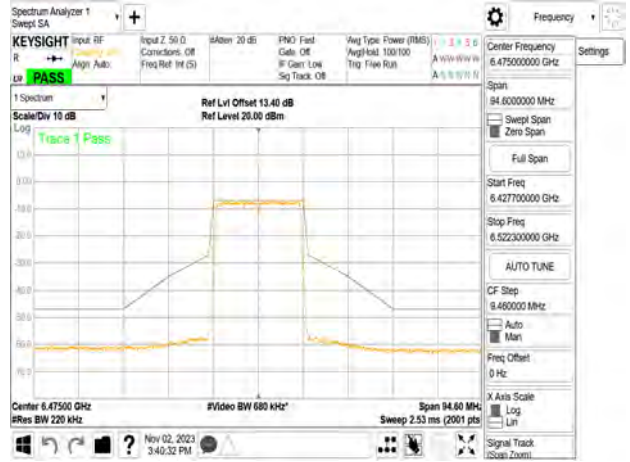
802.11n_20MHz_Chain3_6475MHz
