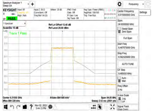
802.11n_20MHz_Chain2_6515MHz
