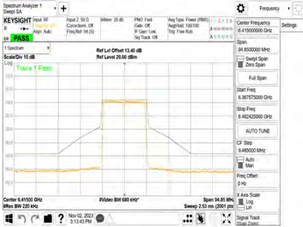
802.11n_20MHz_Chain2_6415MHz
