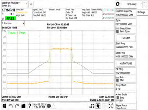
802.11a_20MHz_Chain2_6535MHz
