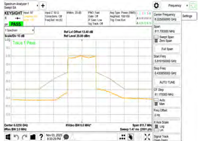
802.11be_160MHz_Chain1_6025MHz
