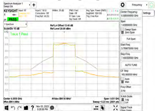
802.11be_320MHz_Chain0_6585MHz
