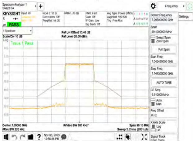
802.11be_20MHz_Chain2_7095MHz
