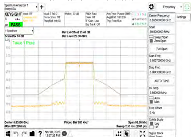
802.11be_20MHz_Chain3_6855MHz
