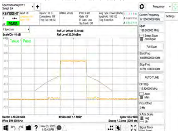
802.11be_40MHz_Chain3_6165MHz
