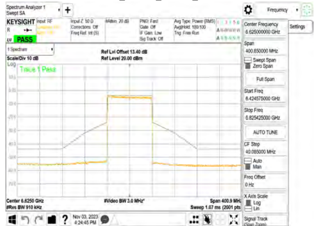
802.11be_80MHz_Chain2_6625MHz
