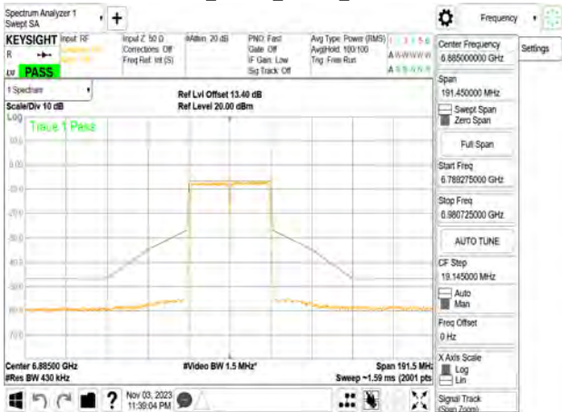
802.11n_40MHz_Chain1_6885MHz
