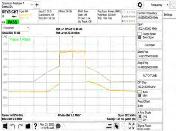
802.11ac_160MHz_Chain0_6025MHz
