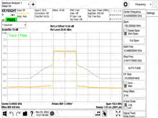
802.11n_40MHz_Chain3_6445MHz
