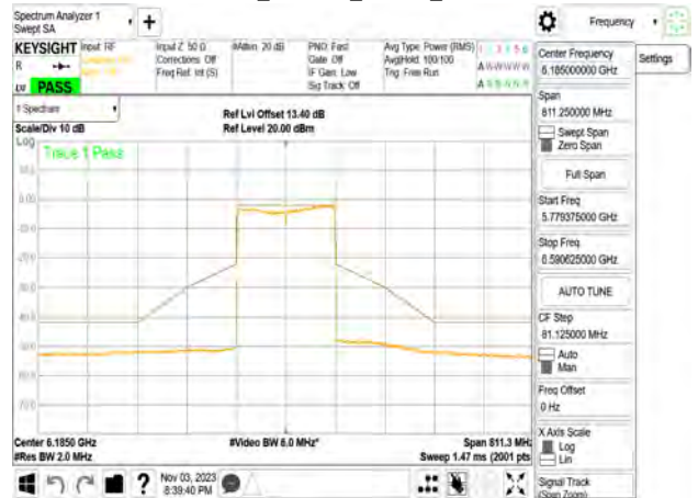
802.11be_160MHz_Chain0_6185MHz
