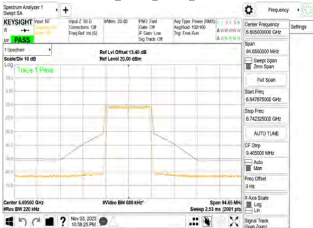
802.11n_20MHz_Chain1_6695MHz
