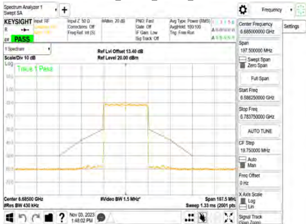
802.11be_40MHz_Chain3_6685MHz
