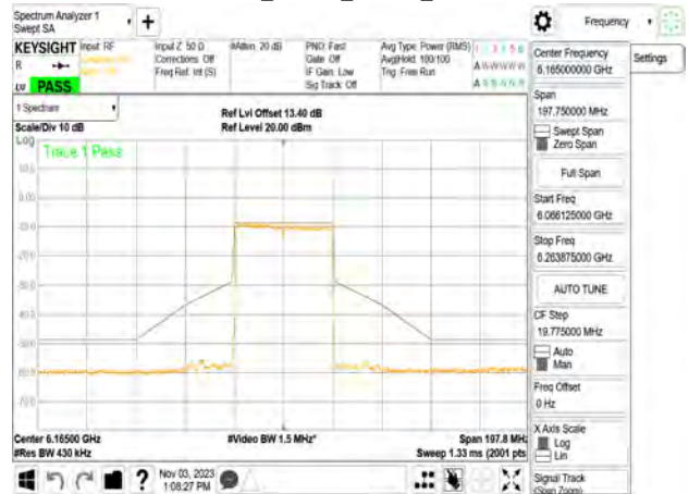
802.11be_40MHz_Chain0_6165MHz
