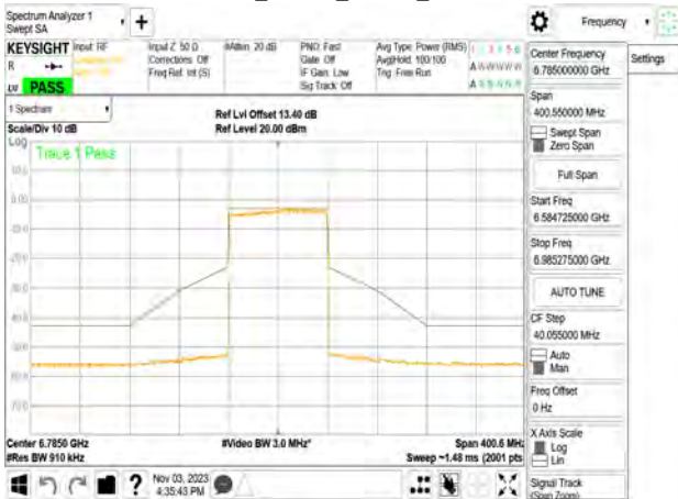
802.11be_80MHz_Chain1_6785MHz
