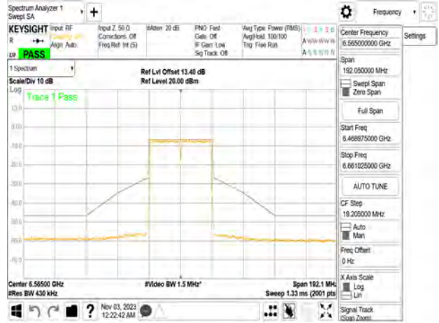
802.11n_40MHz_Chain3_6565MHz
