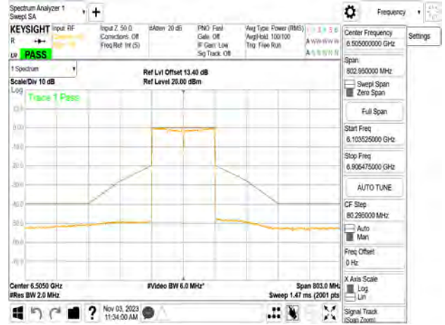
802.11ac_160MHz_Chain0_6505MHz
