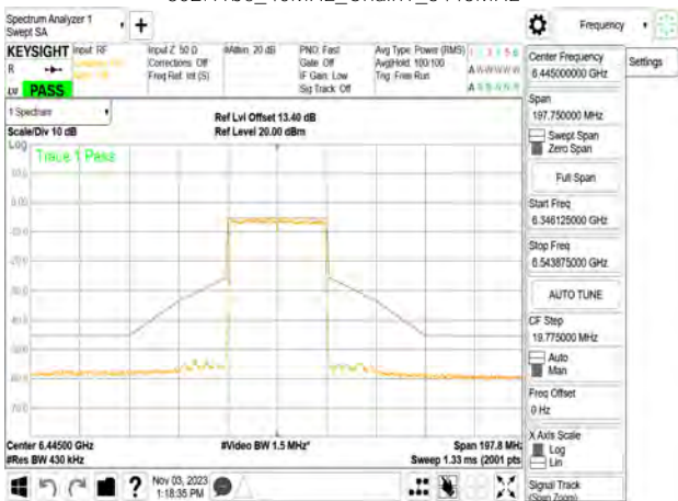
802.11be_40MHz_Chain1_6445MHz
