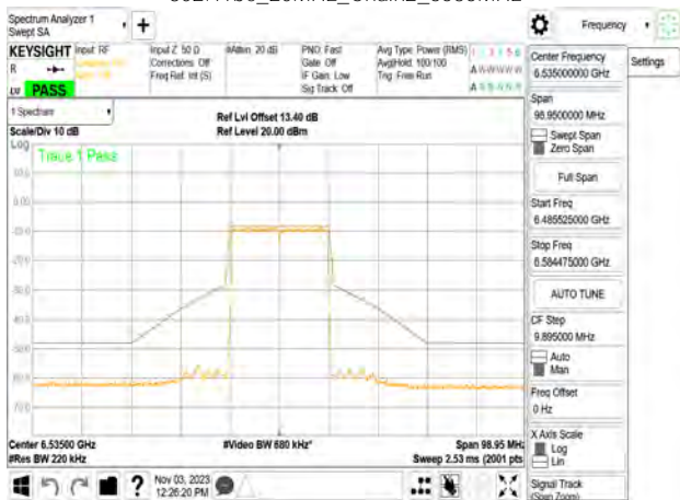
802.11be_20MHz_Chain2_6535MHz
