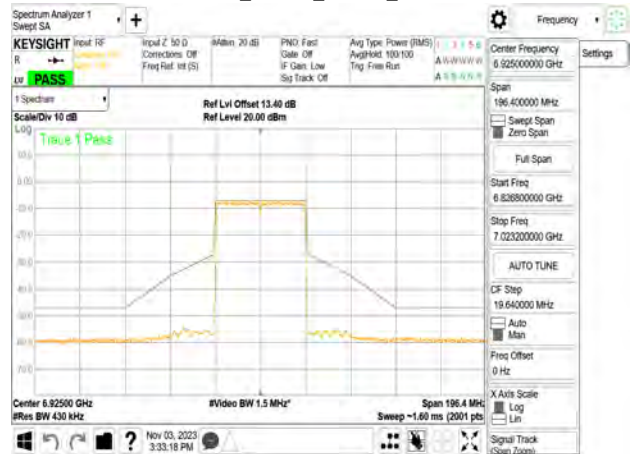
802.11be_40MHz_Chain3_6925MHz
