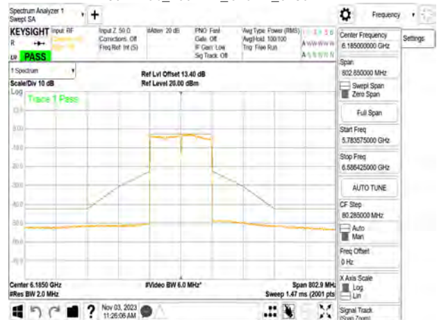
802.11ac_160MHz_Chain2_6185MHz
