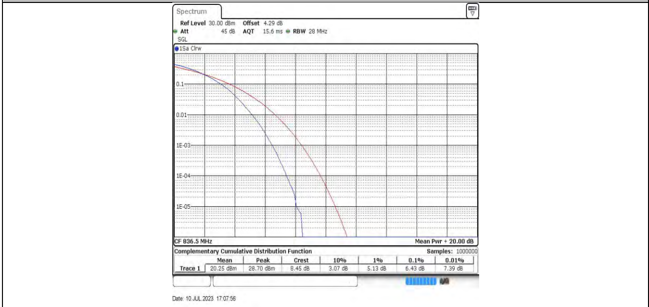
10MHz-20525 64QAM
