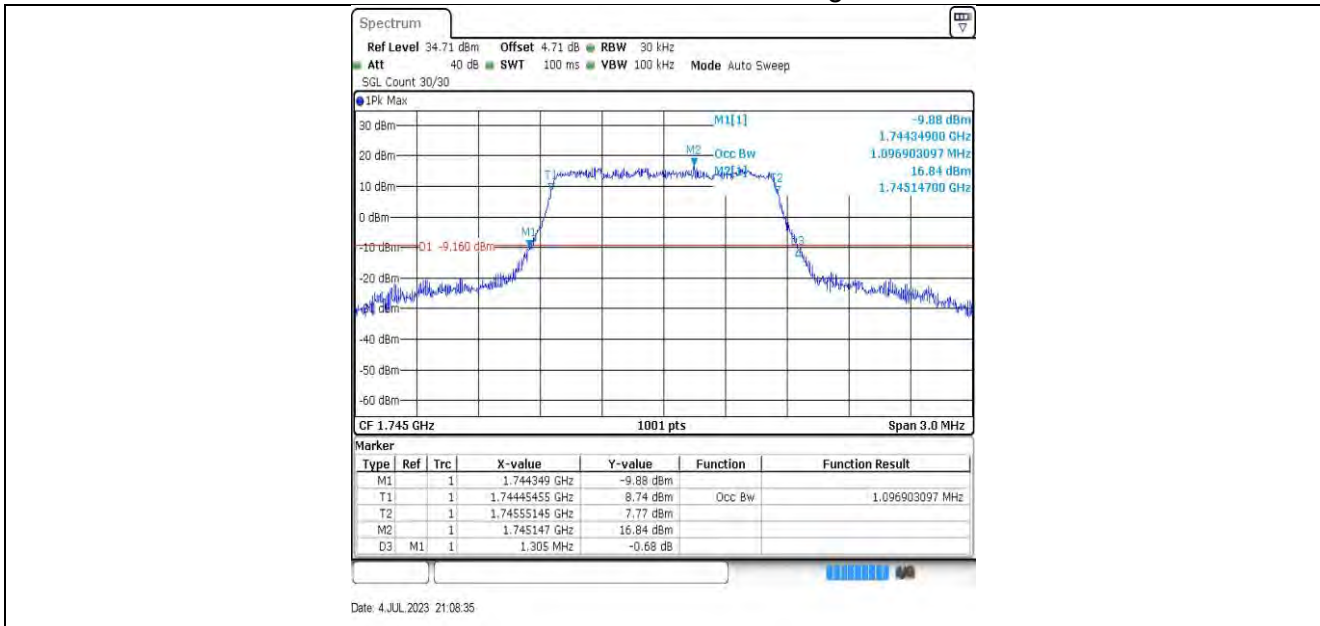
1.4MHz-132322 16QAM
