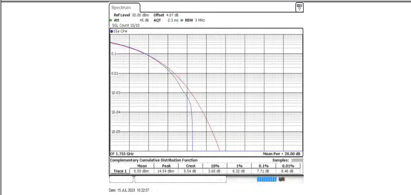
20MHz-20MHz-132323-132521 QPSK-QPSK
