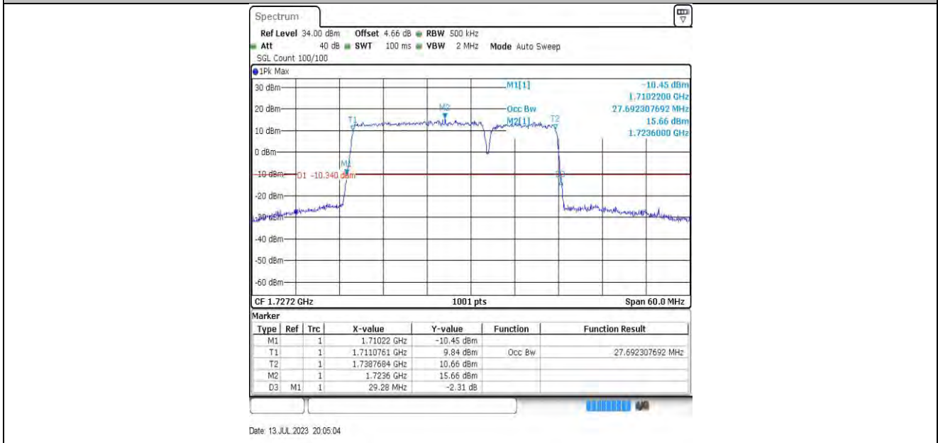
20MHz-10MHz-132072-132216 256QAM-256QAM
