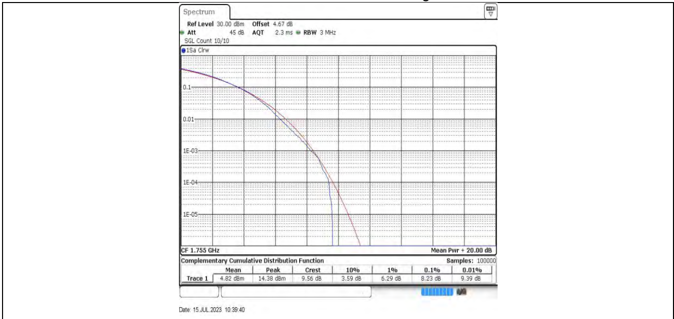
20MHz-20MHz-132323-132521 256QAM-256QAM
