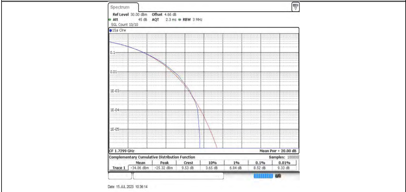
20MHz-20MHz-132072-132270 256QAM-256QAM
