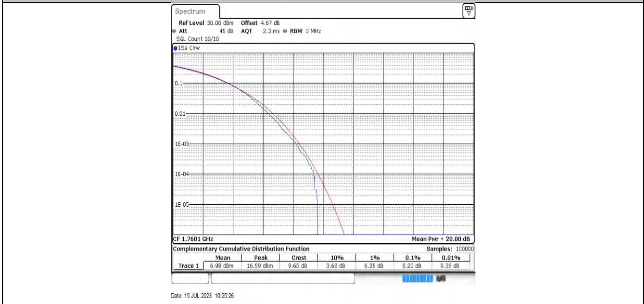
20MHz-20MHz-132374-132572 16QAM-16QAM
