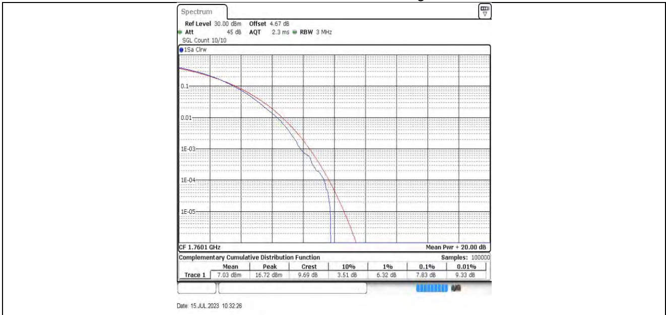
20MHz-20MHz-132374-132572 64QAM-64QAM
