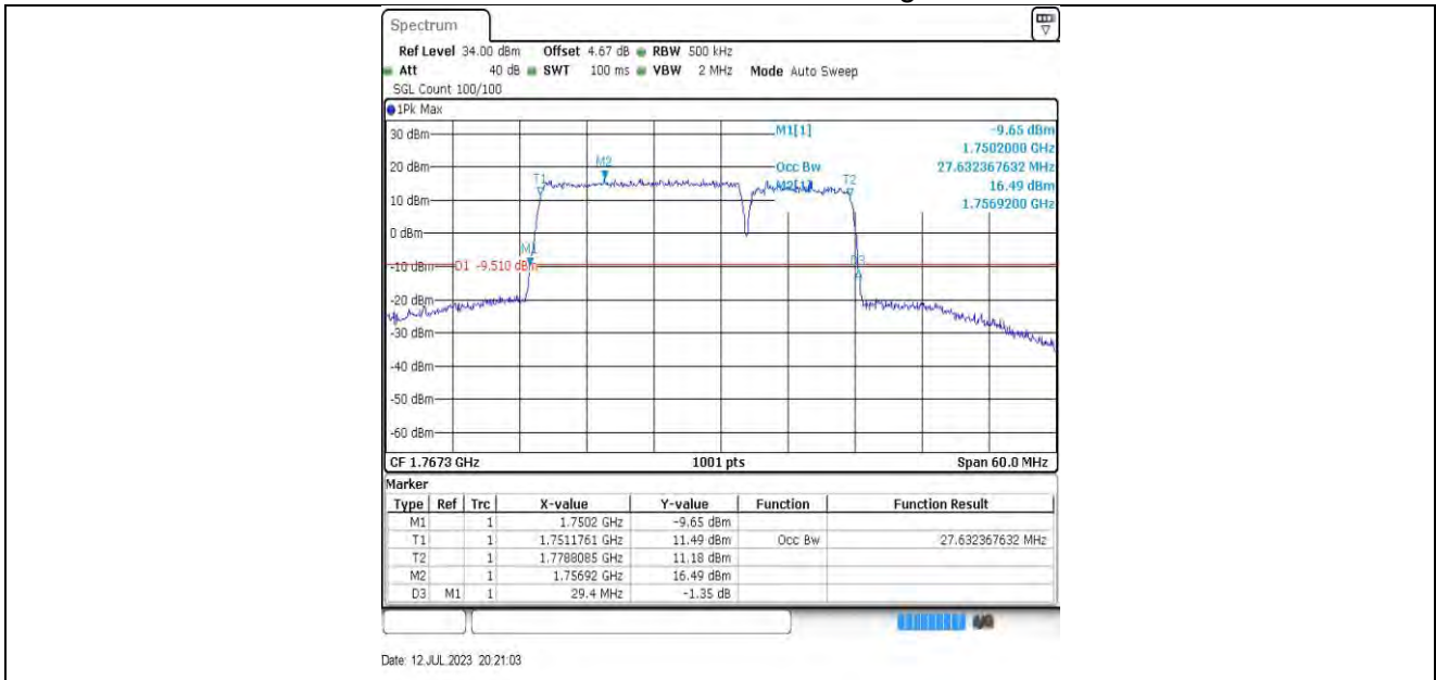
20MHz-10MHz-132473-132617 64QAM-64QAM
