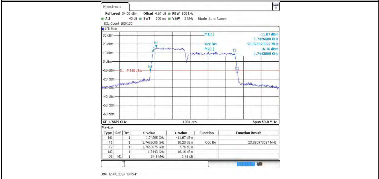
10MHz-15MHz-132351-132471 64QAM-64QAM
