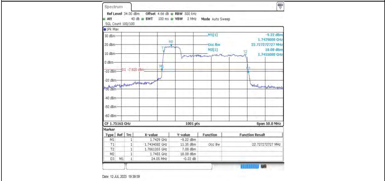
5MHz-20MHz-132330-132447 64QAM-64QAM
