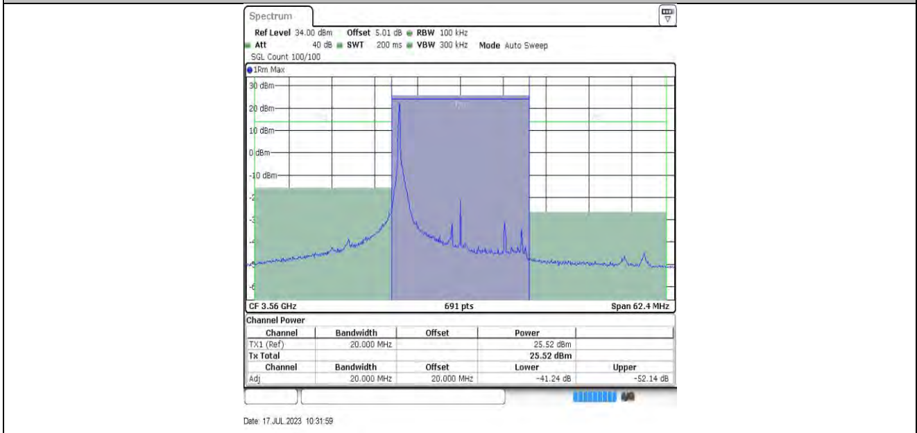
20MHz-55340
