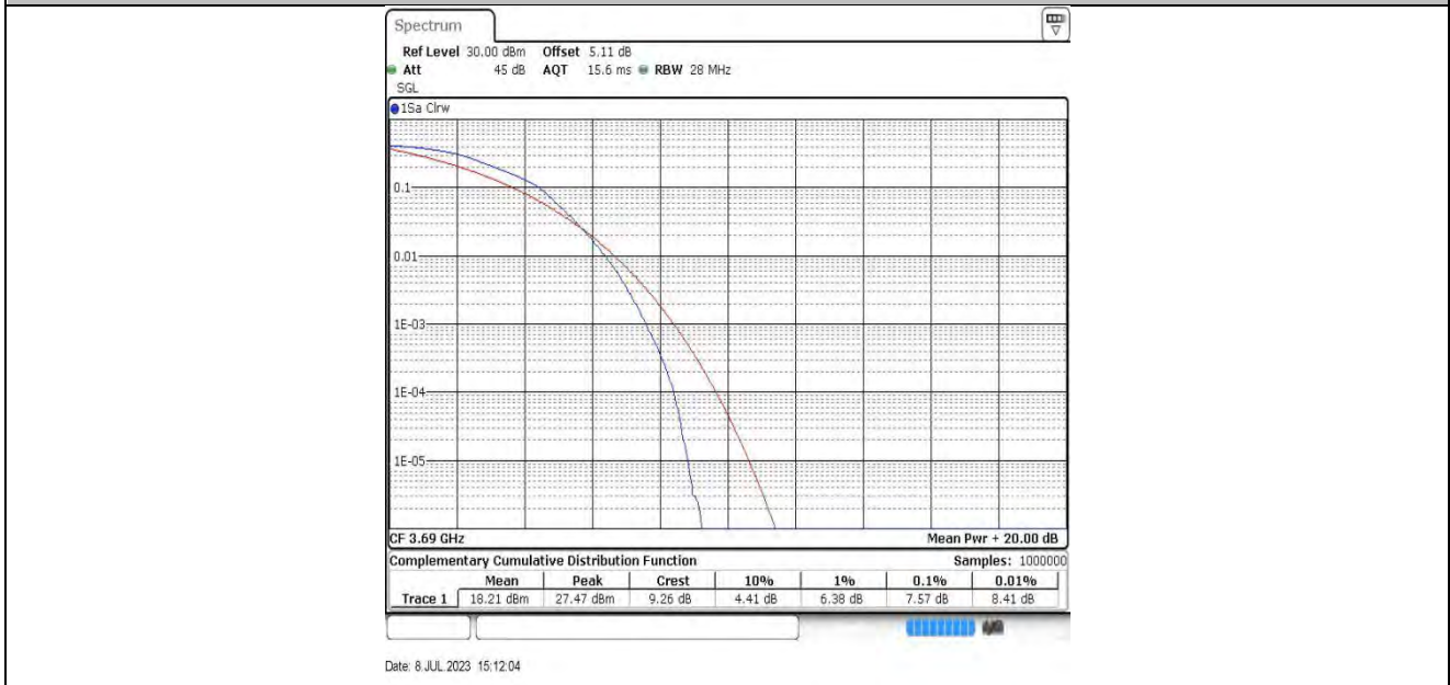
20MHz-56640 16QAM
