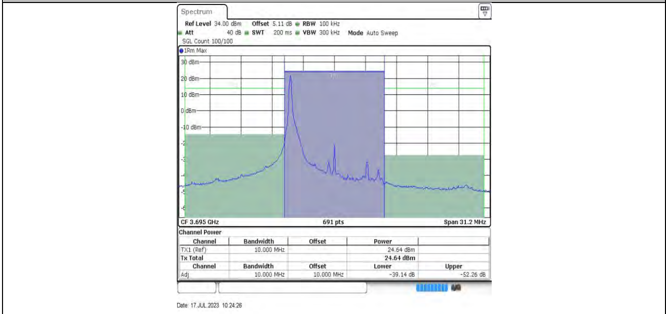
10MHz-56690
