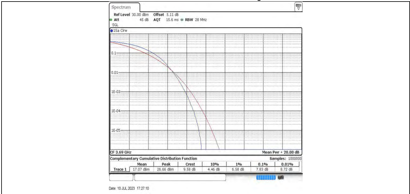
20MHz-56640 64QAM
