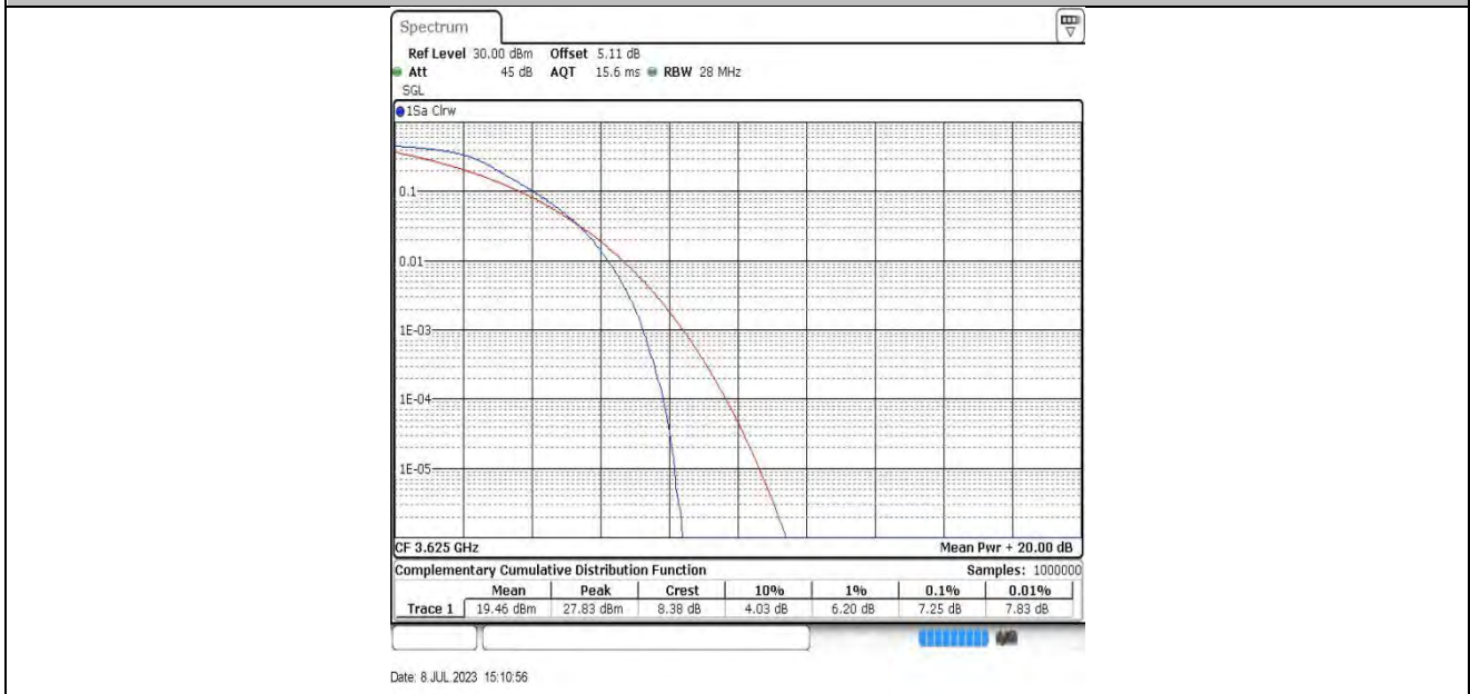
20MHz-55990 QPSK
