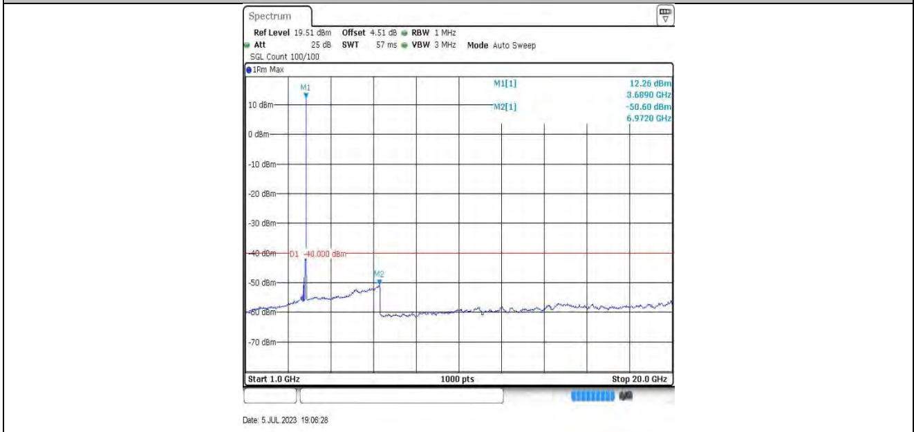
20MHz-56640
