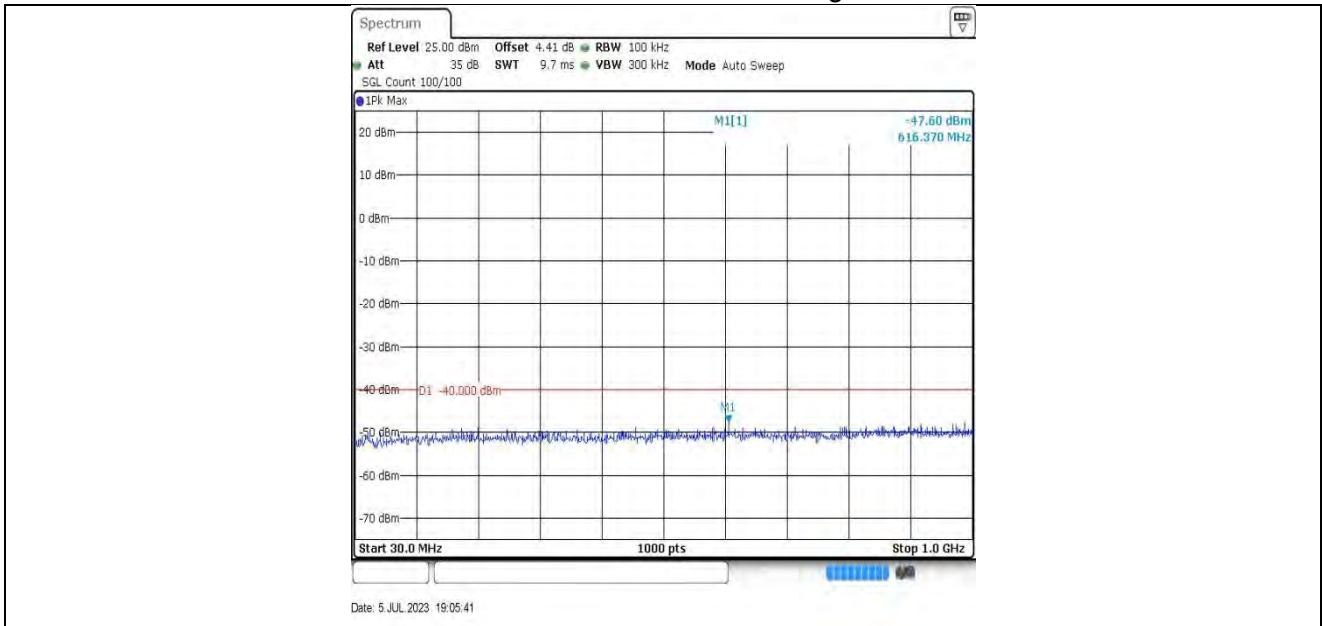
20MHz-56640
