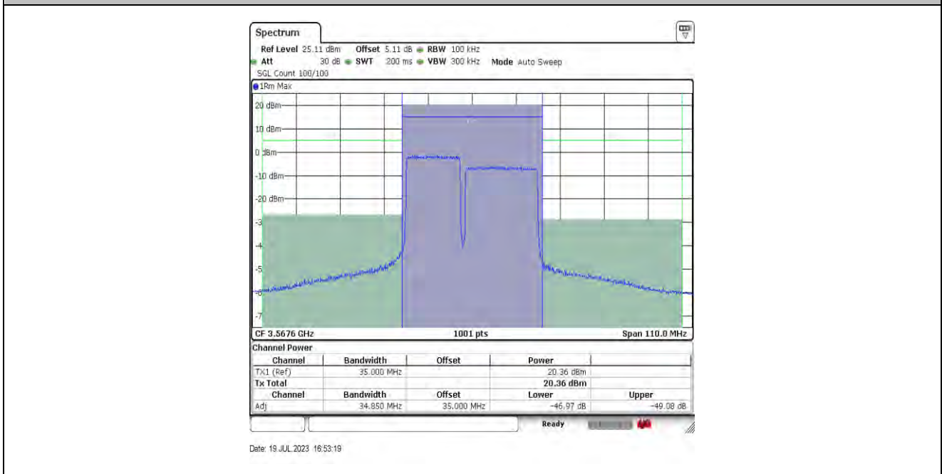
15MHz-20MHz-55318-55489 QPSK-QPSK
