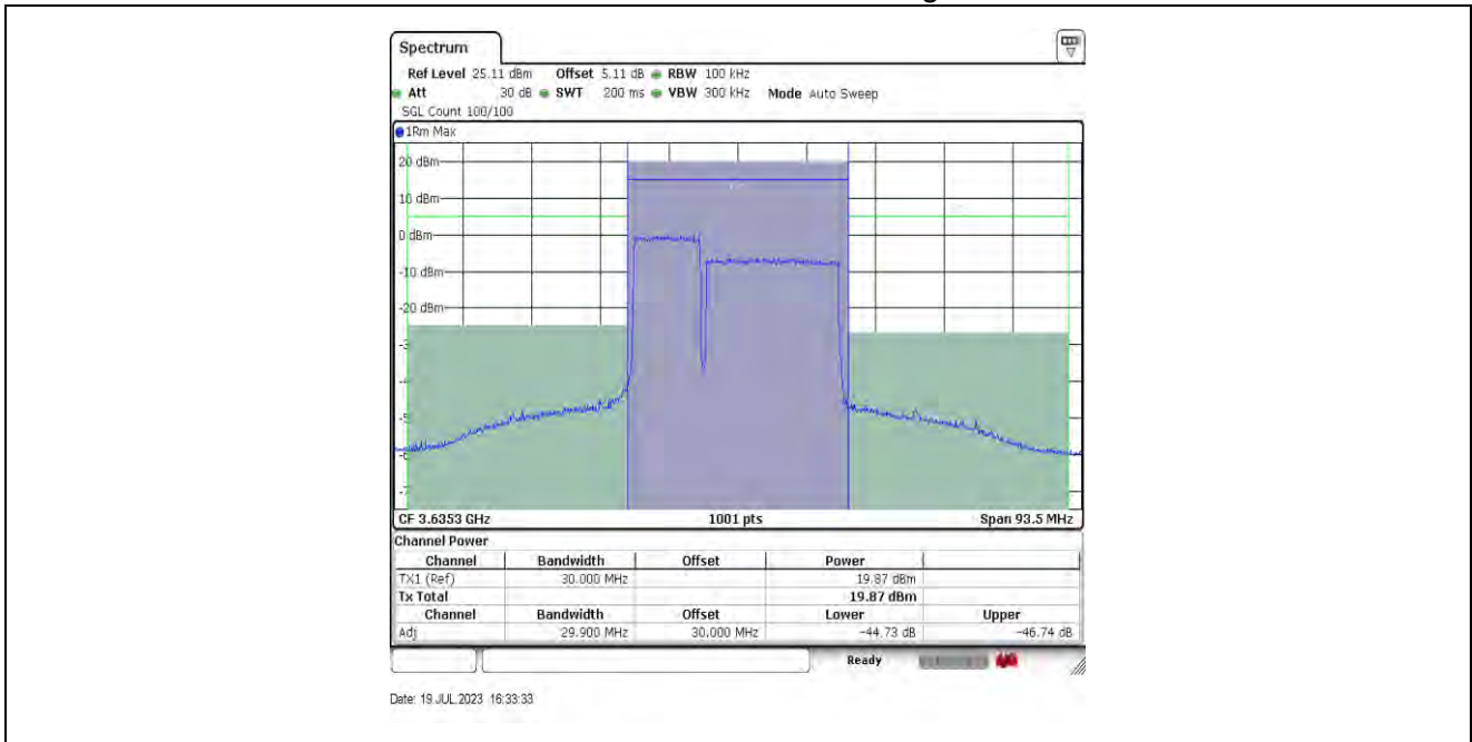
10MHz-20MHz-56496-56640 QPSK-QPSK
