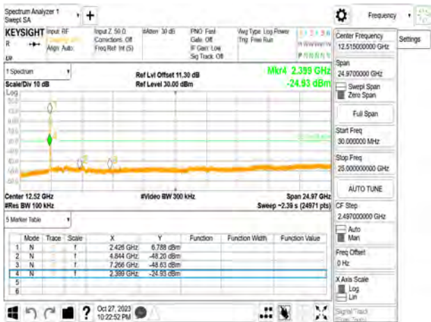
802.11n_40MHz_Chain2_2437MHz
