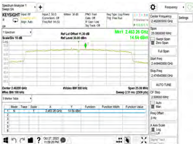
802.11be_20MHz_Chain0_2462MHz
