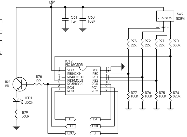
PIC16C505 16個CH切換 含送DISPLAY資料輸出, 預計使用內部OSC=4MHZ
