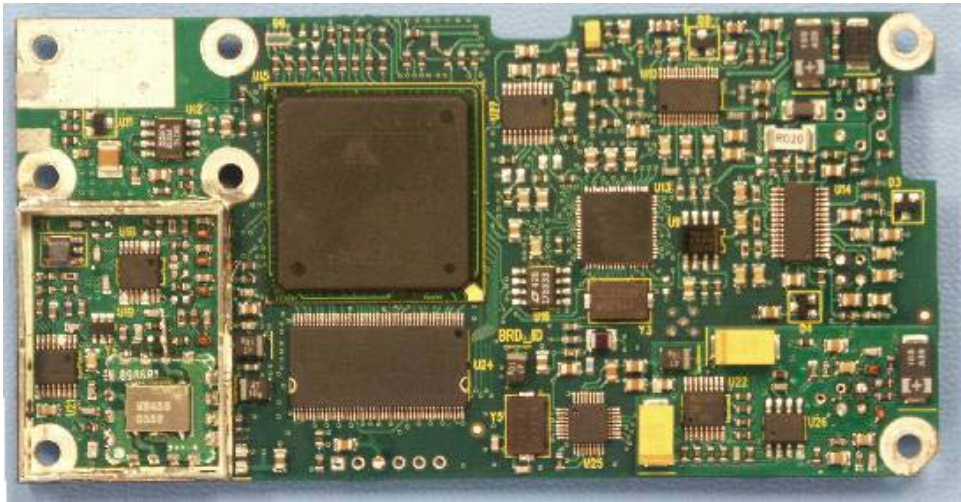
PCB Bottom
