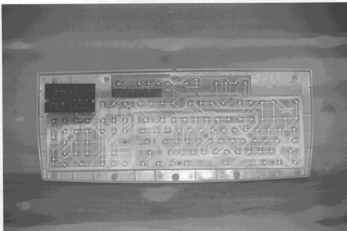
EUT Inside View(2)
