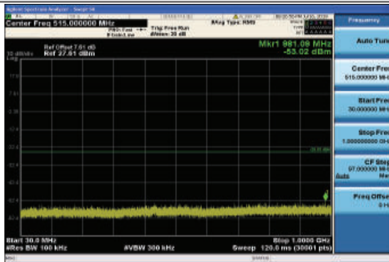
Band41-5MHz-QPSK-41215-1RB#0-30~1000MHz
