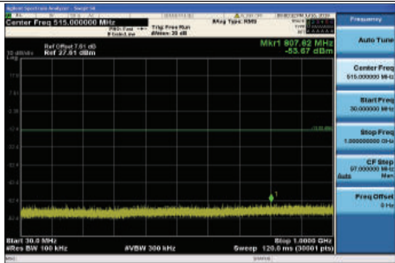
Band25-1.4MHz-QPSK-26365-1RB#0-30~1000MHz
