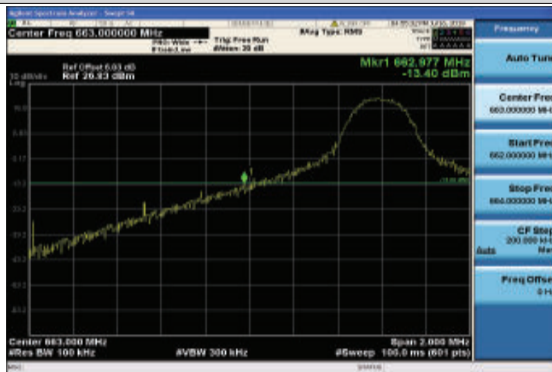
Band71-10MHz-QPSK-133172-1RB#0
