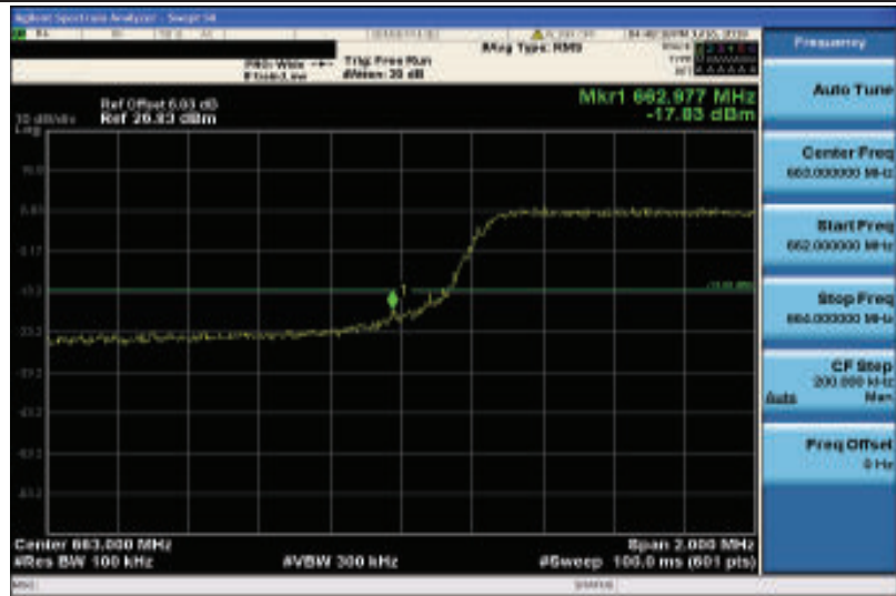
Band71-5MHz-QPSK-133147-25RB#0
