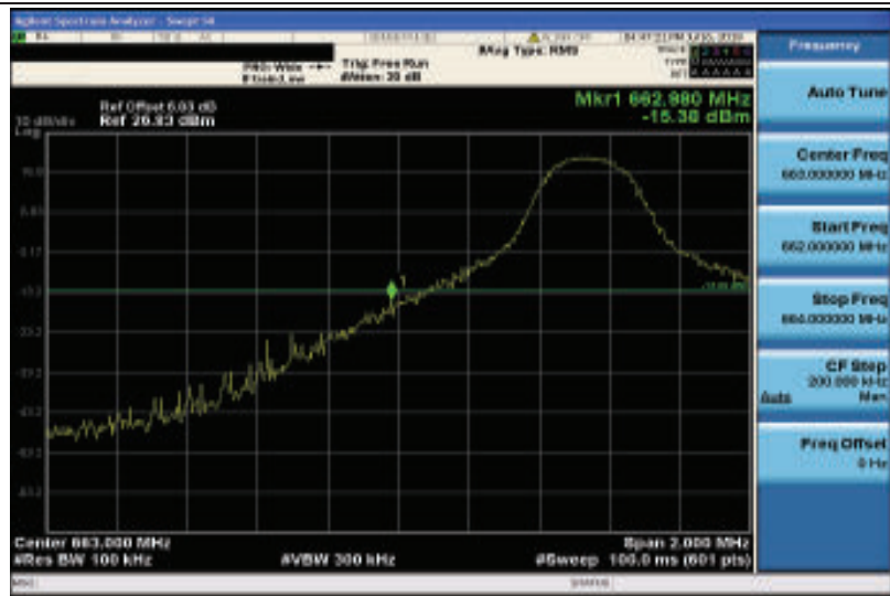
Band71-5MHz-QPSK-133147-1RB#0
