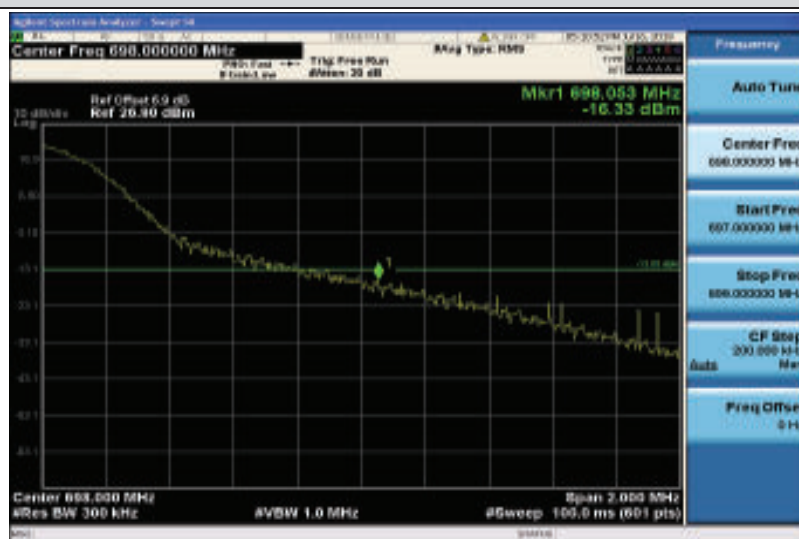
Band71-20MHz-QPSK-133372-1RB#99
