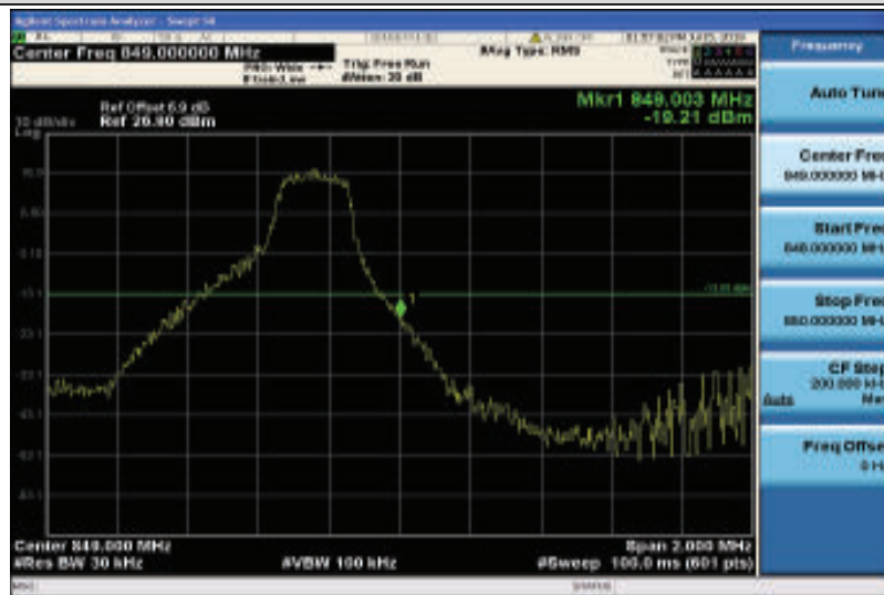
Band5-3MHz-QPSK-20635-1RB#14
