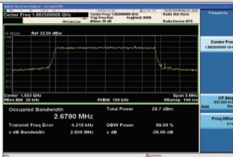
Band25-3MHz-QPSK-26365-15RB#0-2.6790
