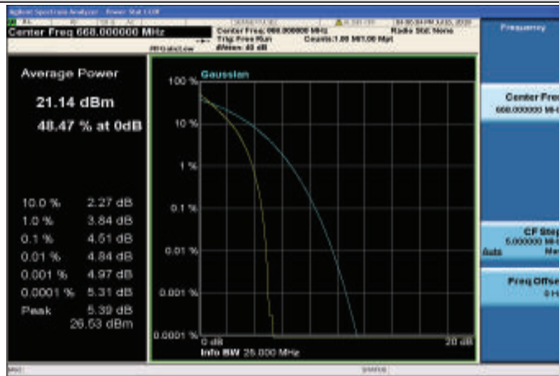
Band71-10MHz-QPSK-133172-50RB#0
