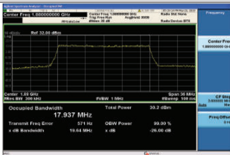
Band2-20MHz-QPSK-18900-100RB#0-17.937
