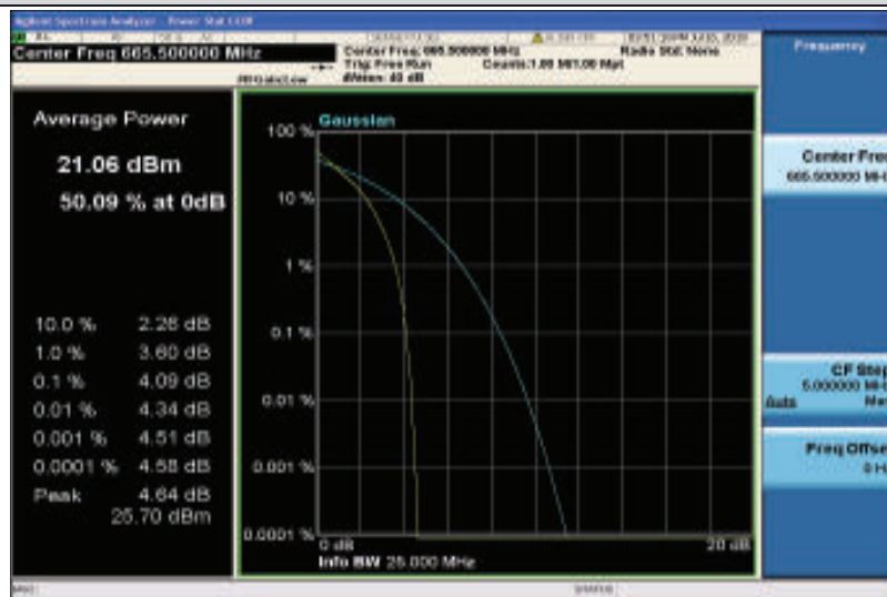
Band71-5MHz-QPSK-133147-25RB#0
