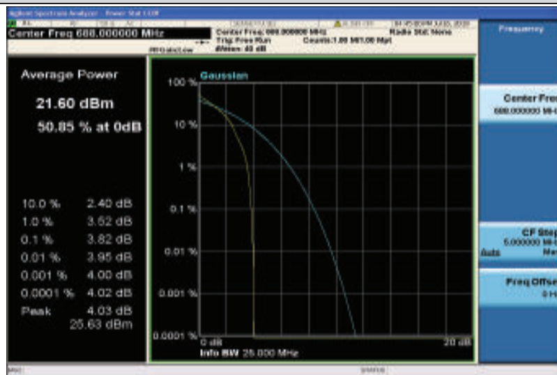
Band71-20MHz-QPSK-133372-1RB#0
