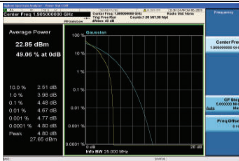
Band25-20MHz-QPSK-26590-1RB#0
