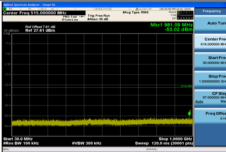
Band41-5MHz-QPSK-41215-1RB#0-30~1000MHz
