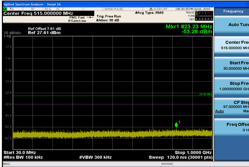
Band41-10MHz-QPSK-40290-1RB#0-30~1000MHz
