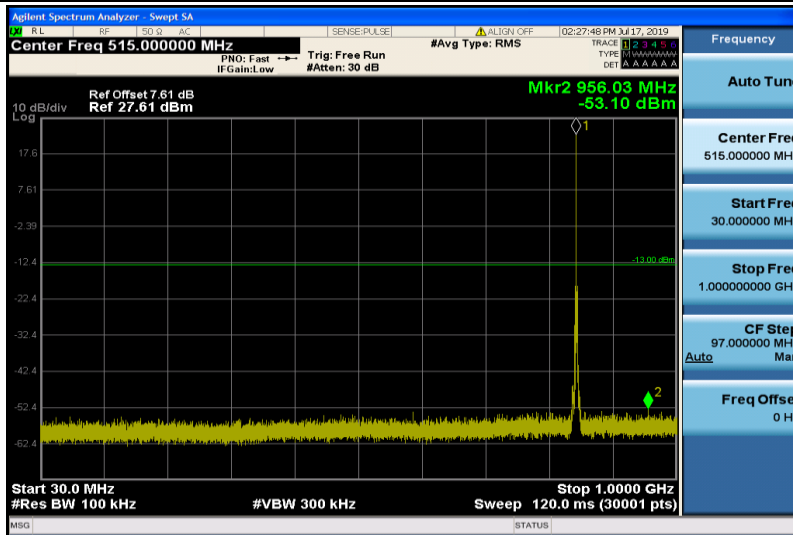
Band26-3MHz-QPSK-27025-1RB#0-30~1000MHz
