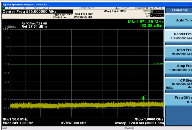
Band25-20MHz-QPSK-26365-1RB#0-30~1000MHz
