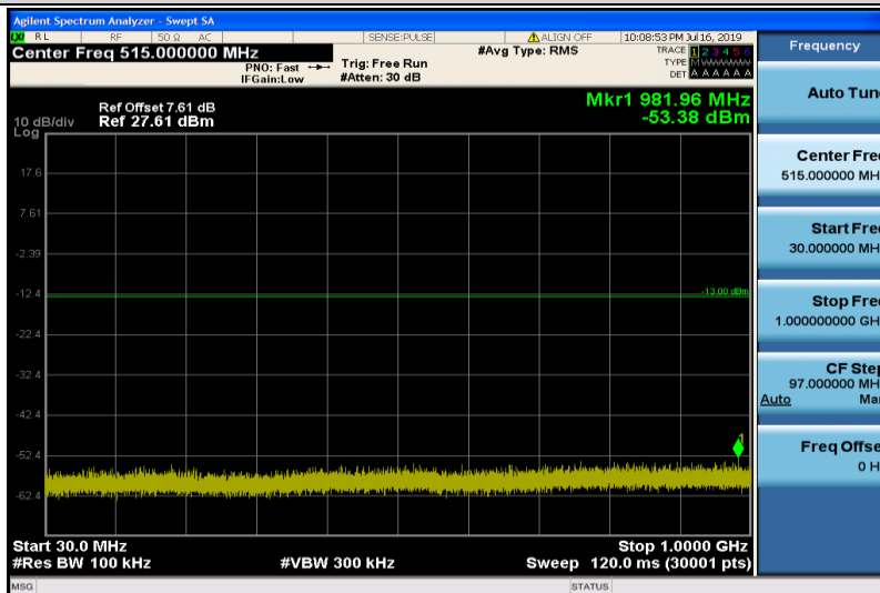
Band25-20MHz-16QAM-26365-1RB#0-30~1000MHz
