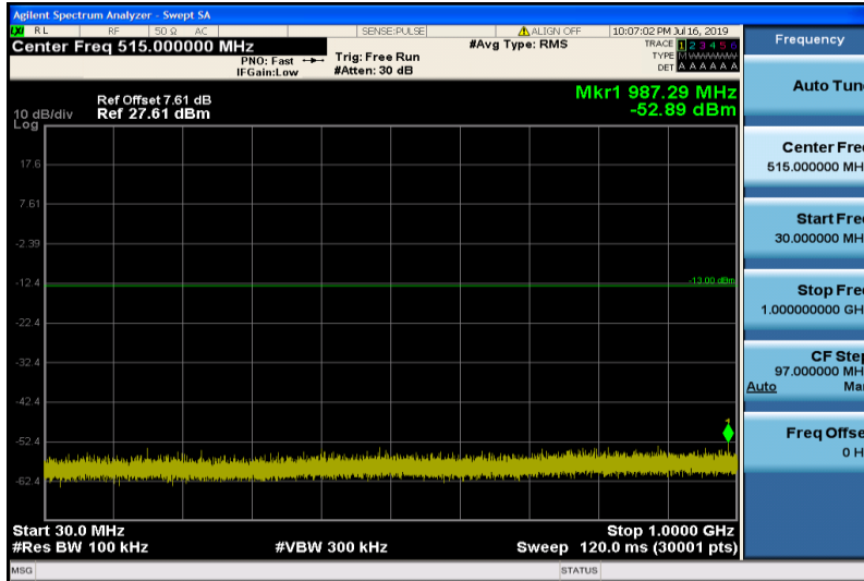
Band25-20MHz-QPSK-26140-1RB#0-30~1000MHz
