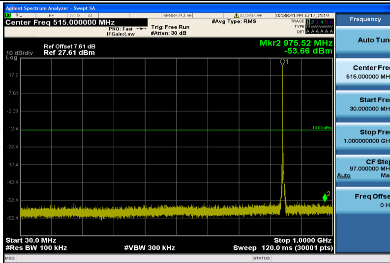
Band26-5MHz-QPSK-27015-1RB#0-30~1000MHz
