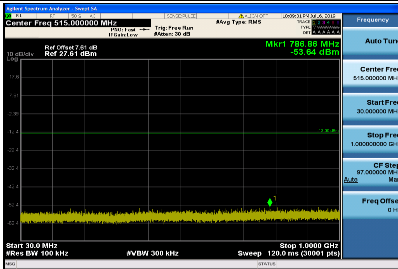
Band25-20MHz-QPSK-26590-1RB#0-30~1000MHz
