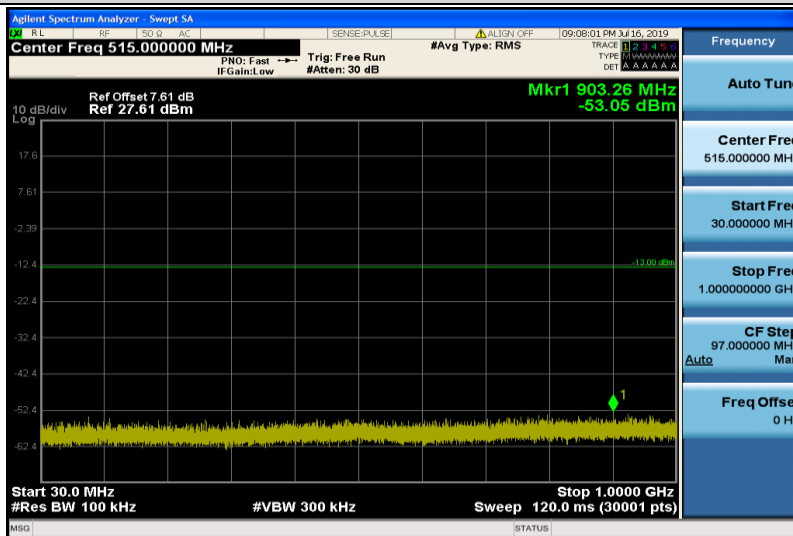
Band25-3MHz-QPSK-26365-1RB#0-30~1000MHz
