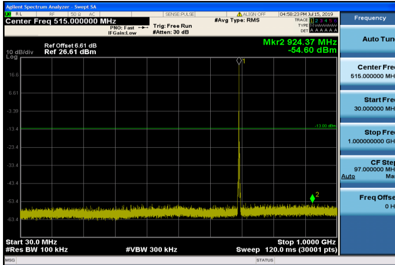
Band12-1.4MHz-QPSK-23017-1RB#0-Range1:30~1000MHz
