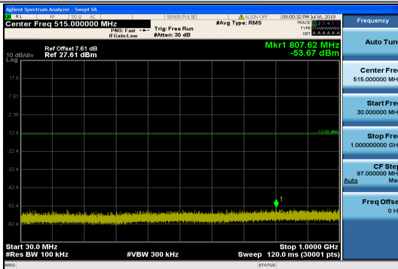
Band25-1.4MHz-QPSK-26365-1RB#0-30~1000MHz
