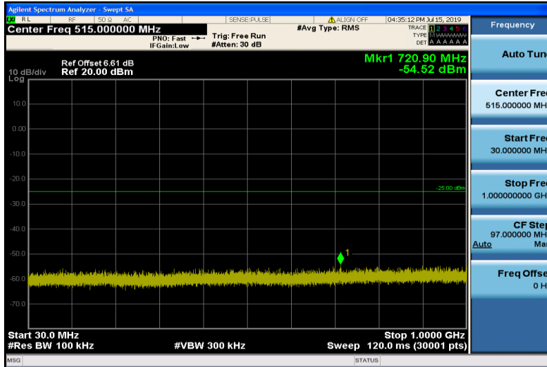
Band7-10MHz-QPSK-20800-1RB#0-Range1:30~1000MHz
