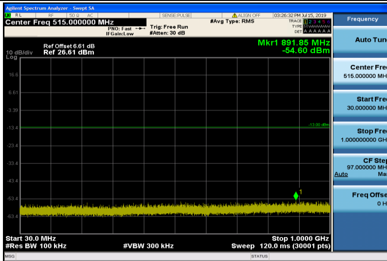
Band4-1.4MHz-QPSK-20393-1RB#0-Range1:30~1000MHz
