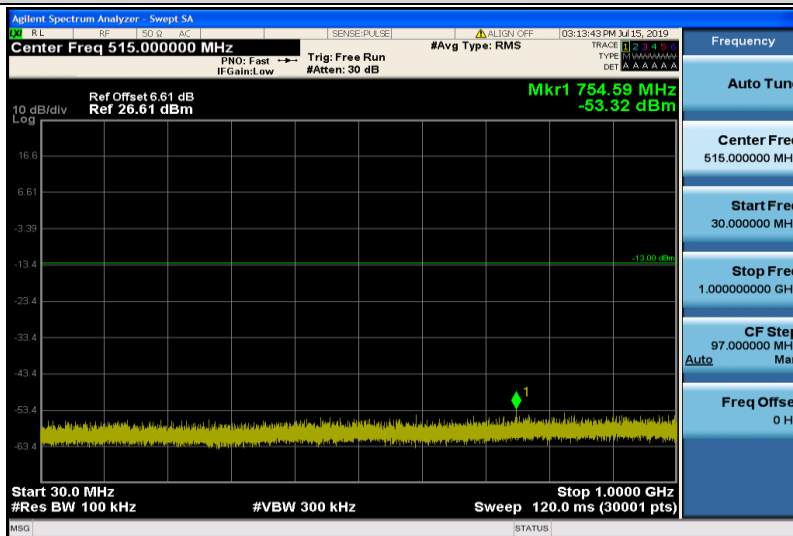
Band2-20MHz-QPSK-18900-1RB#0-Range1:30~1000MHz
