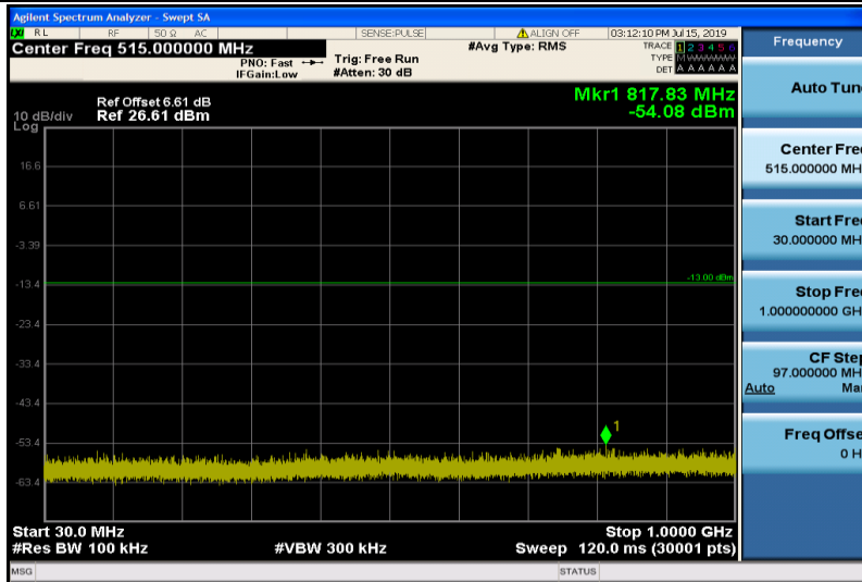
Band2-20MHz-QPSK-18700-1RB#0-Range1:30~1000MHz
