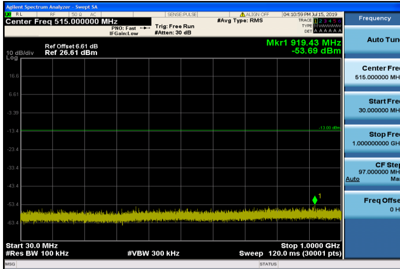
Band4-10MHz-QPSK-20000-1RB#0-Range1:30~1000MHz
