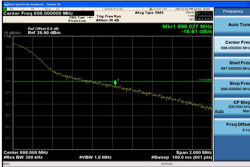
Band71-20MHz-16QAM-133372-1RB#99
