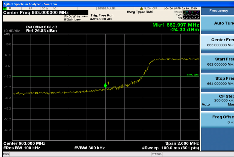
Band71-10MHz-QPSK-133172-50RB#0
