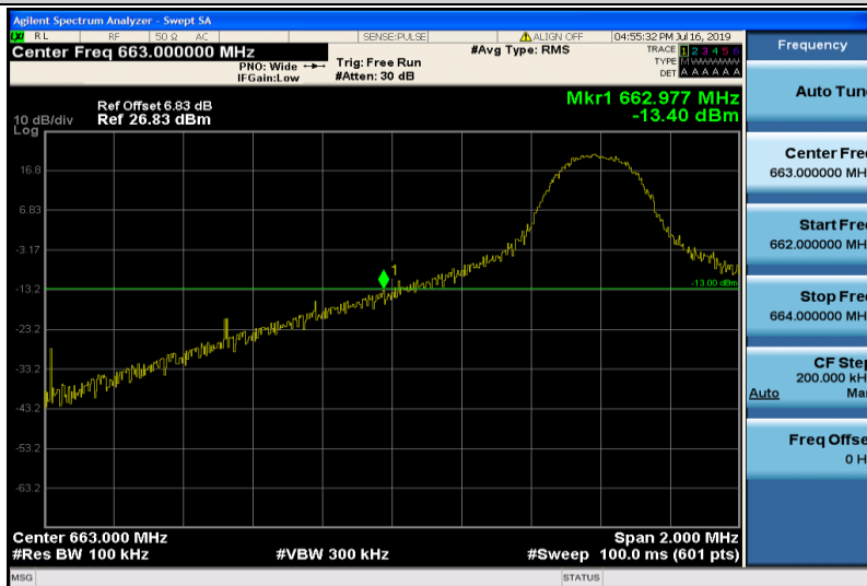
Band71-10MHz-QPSK-133172-1RB#0
