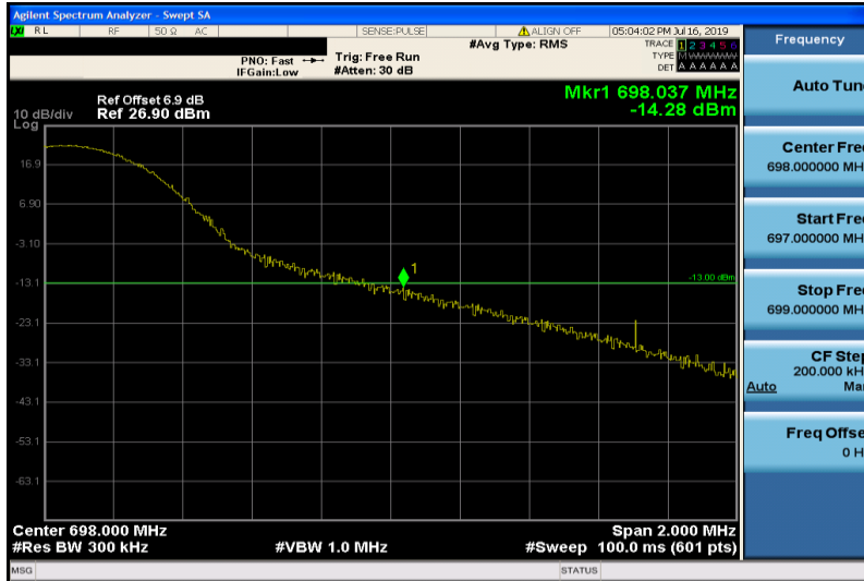
Band71-15MHz-QPSK-133397-1RB#74
