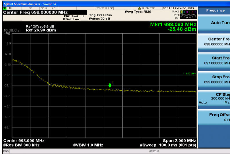
Band71-20MHz-QPSK-133372-100RB#0
