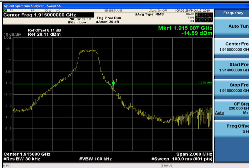
Band25-3MHz-QPSK-26675-1RB#14
