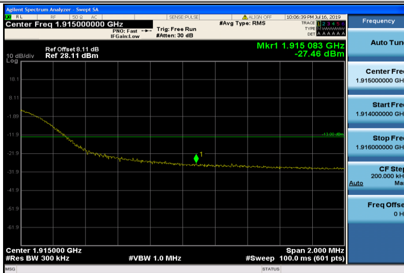
Band25-20MHz-QPSK-26590-100RB#0
