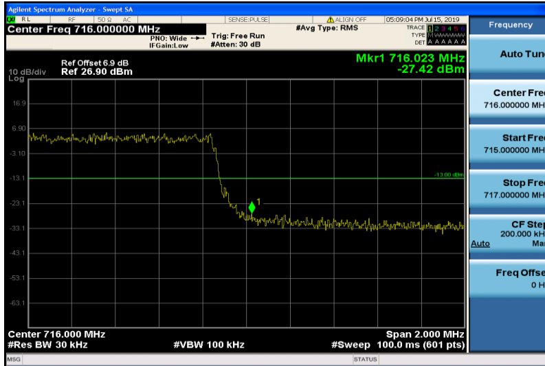
Band12-3MHz-QPSK-23165-15RB#0
