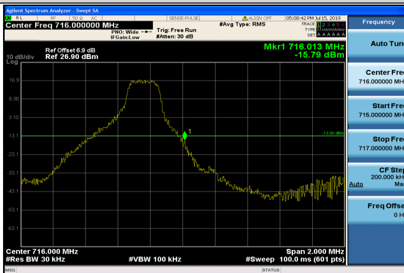
Band12-3MHz-QPSK-23165-1RB#14
