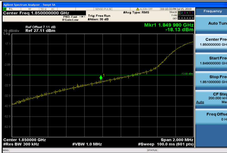
Band2-20MHz-QPSK-18700-1RB#0
