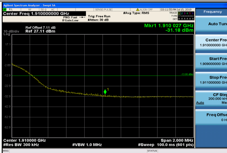
Band2-20MHz-16QAM-19100-100RB#0
