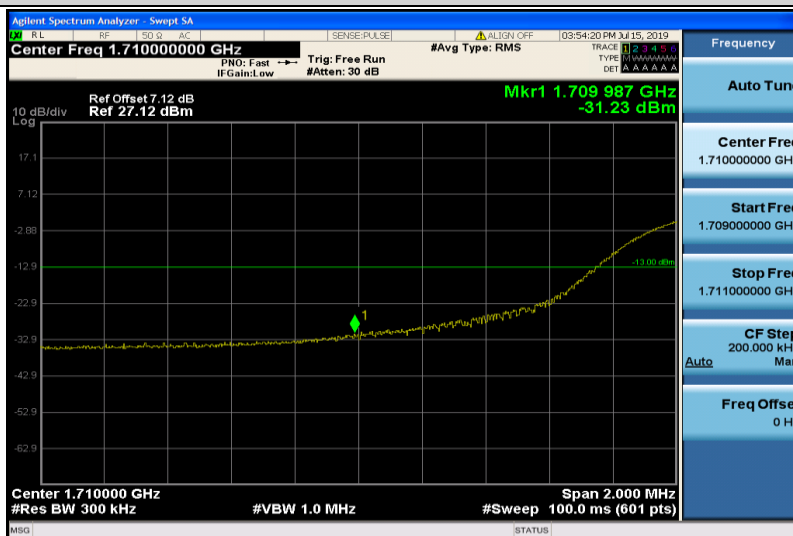
Band4-20MHz-QPSK-20050-100RB#0
