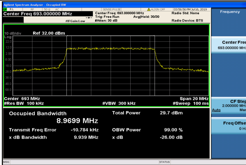
Band71-10MHz-QPSK-133422-50RB#0-8.9699
