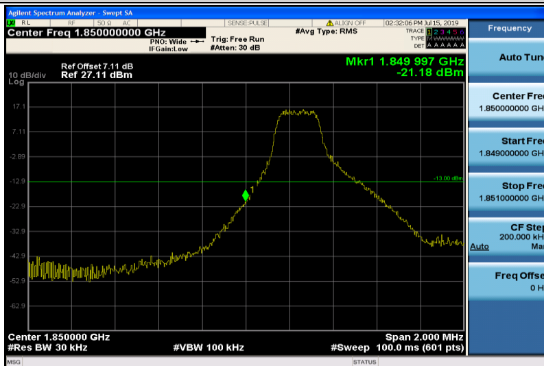
Band2-3MHz-QPSK-18615-1RB#0
