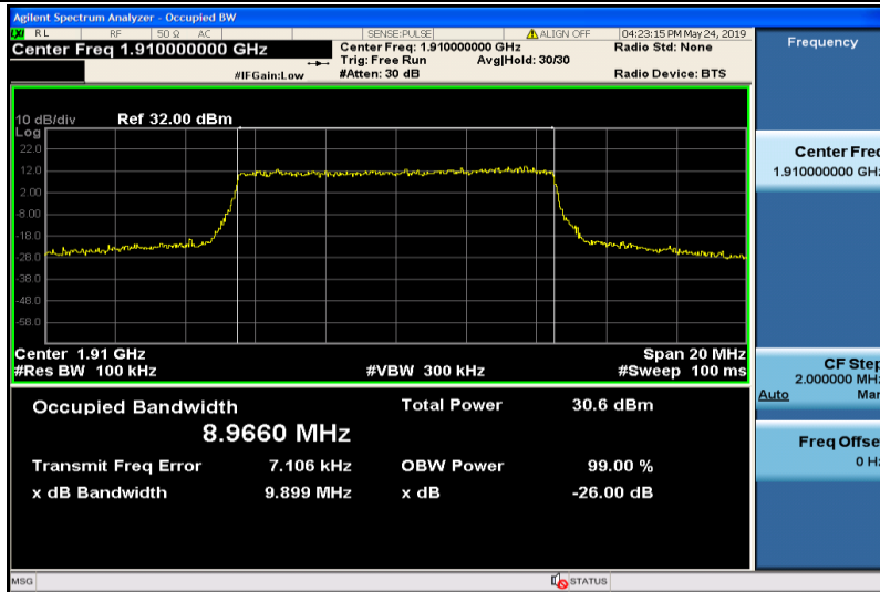
Band25-10MHz-QPSK-26640-50RB#0-8.9660
