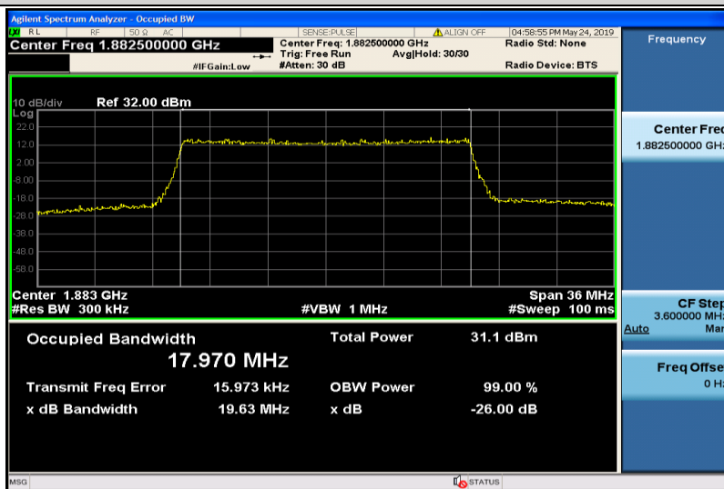
Band25-20MHz-QPSK-26365-100RB#0-17.970
