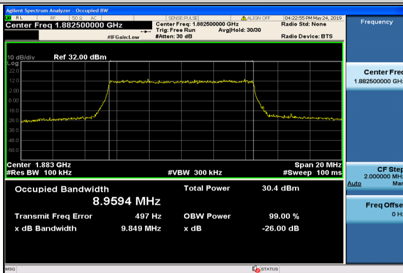
Band25-10MHz-QPSK-26365-50RB#0-8.9594
