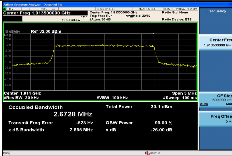
Band25-3MHz-QPSK-26675-15RB#0-2.6728
