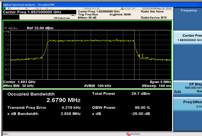
Band25-3MHz-QPSK-26365-15RB#0-2.6790
