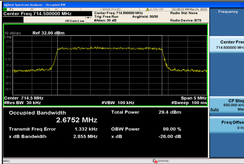
Band12-3MHz-QPSK-23165-15RB#0-2.6752
