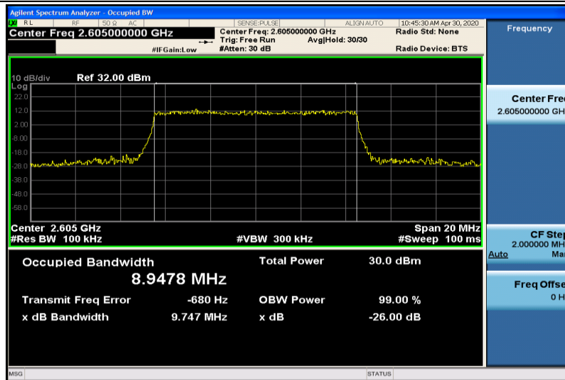
Band41-10MHz-QPSK-40740-50RB#0-8.9478
