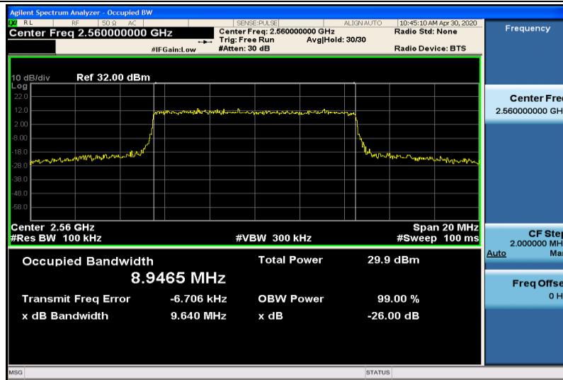
Band41-10MHz-QPSK-40290-50RB#0-8.9465
