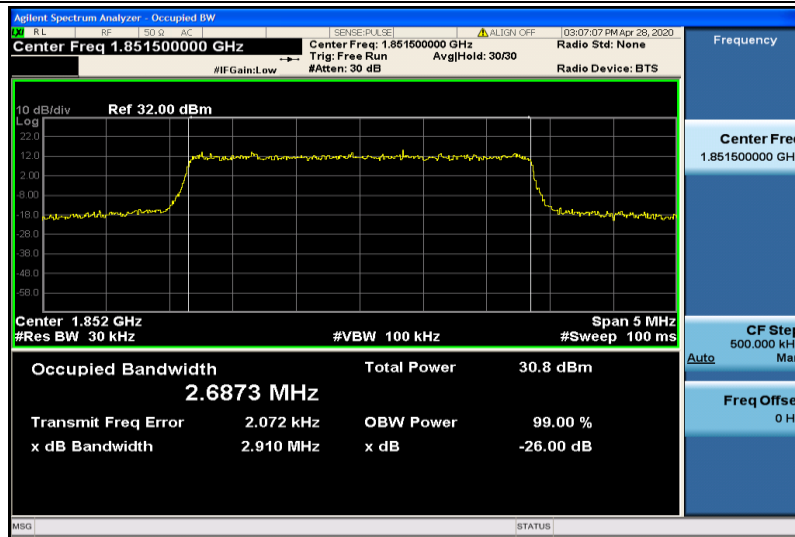
Band2-3MHz-QPSK-18615-15RB#0-2.6873
