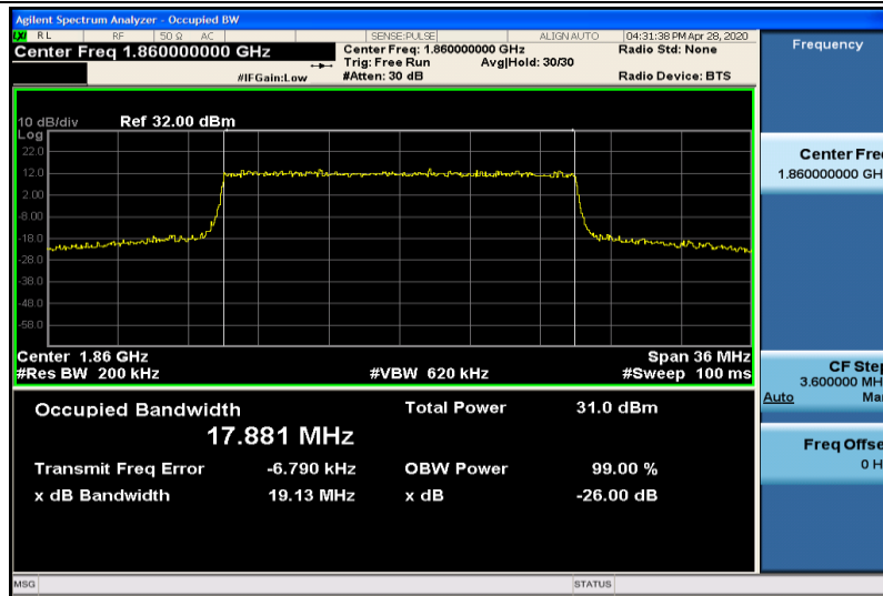
Band2-20MHz-QPSK-18700-100RB#0-17.881
