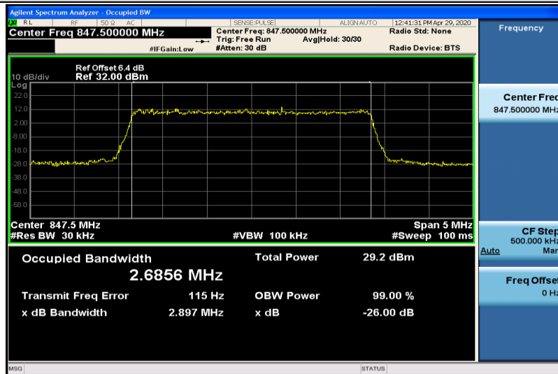
Band5-3MHz-QPSK-20635-15RB#0-2.6856
