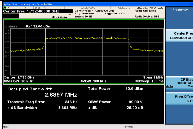
Band4-3MHz-QPSK-20175-15RB#0-2.6897
