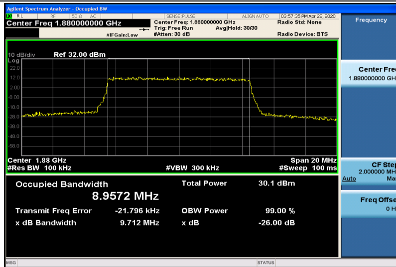
Band2-10MHz-QPSK-18900-50RB#0-8.9572
