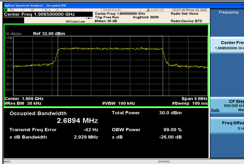
Band2-3MHz-QPSK-19185-15RB#0-2.6894
