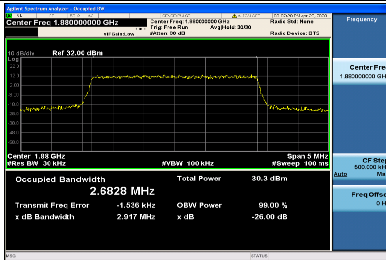
Band2-3MHz-QPSK-18900-15RB#0-2.6828
