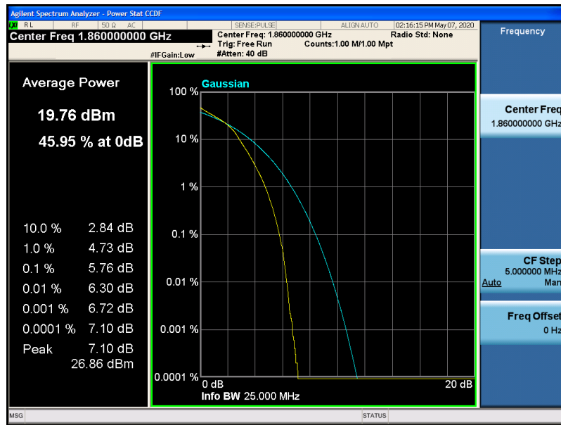
Band2-20MHz-16QAM-18700-100RB#0
