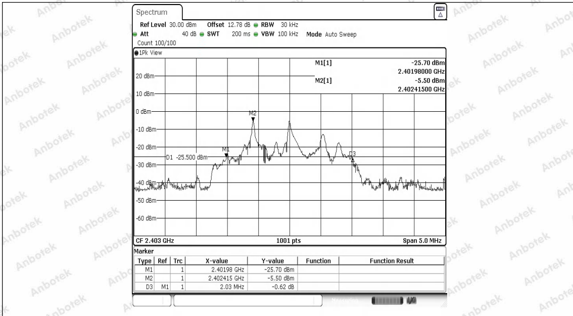
2.4G-Ant1-2403
