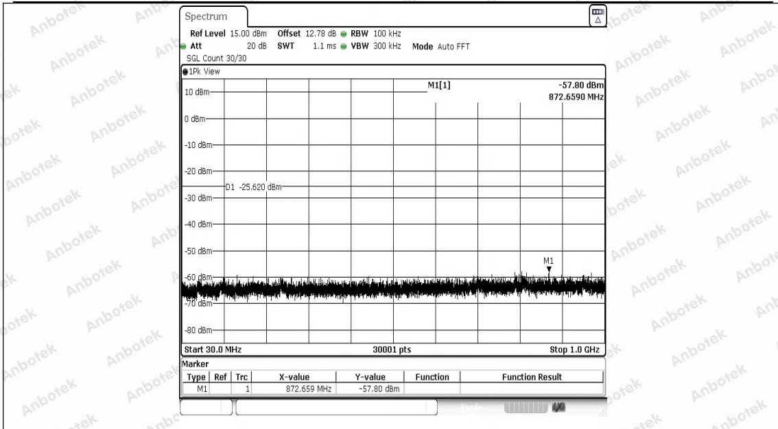
2.4G-Ant1-2441-30~1000-PASS
