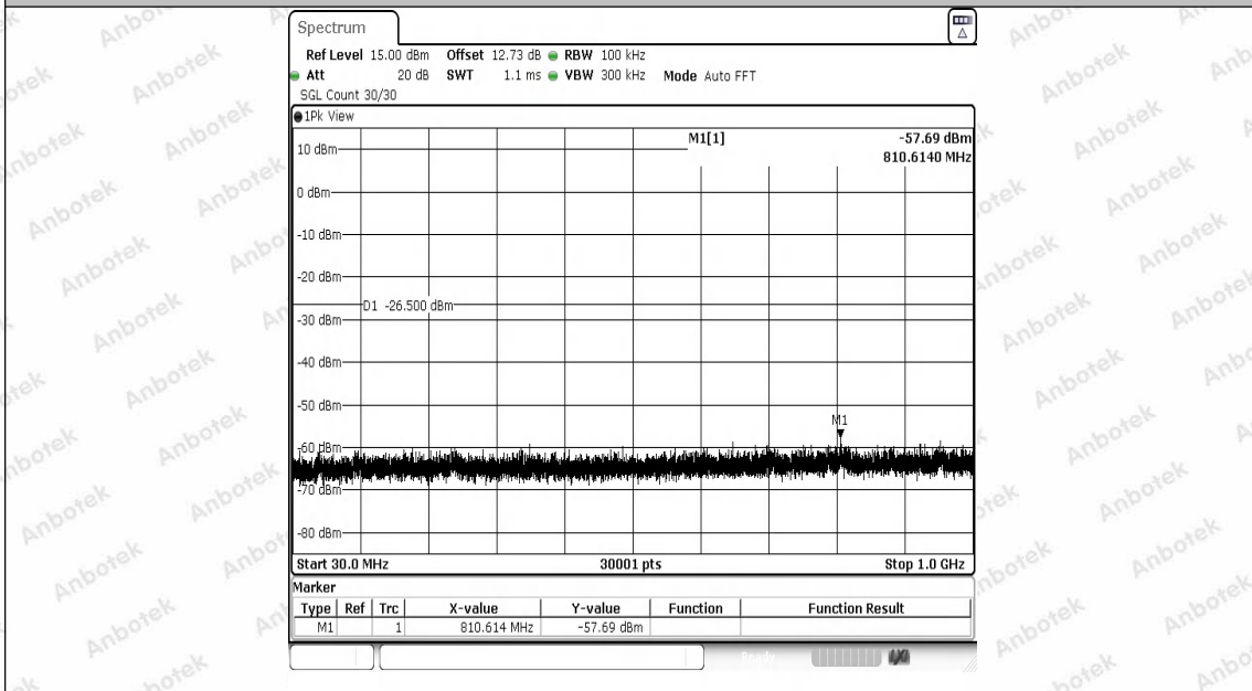
2.4G-Ant1-2479-30~1000-PASS
