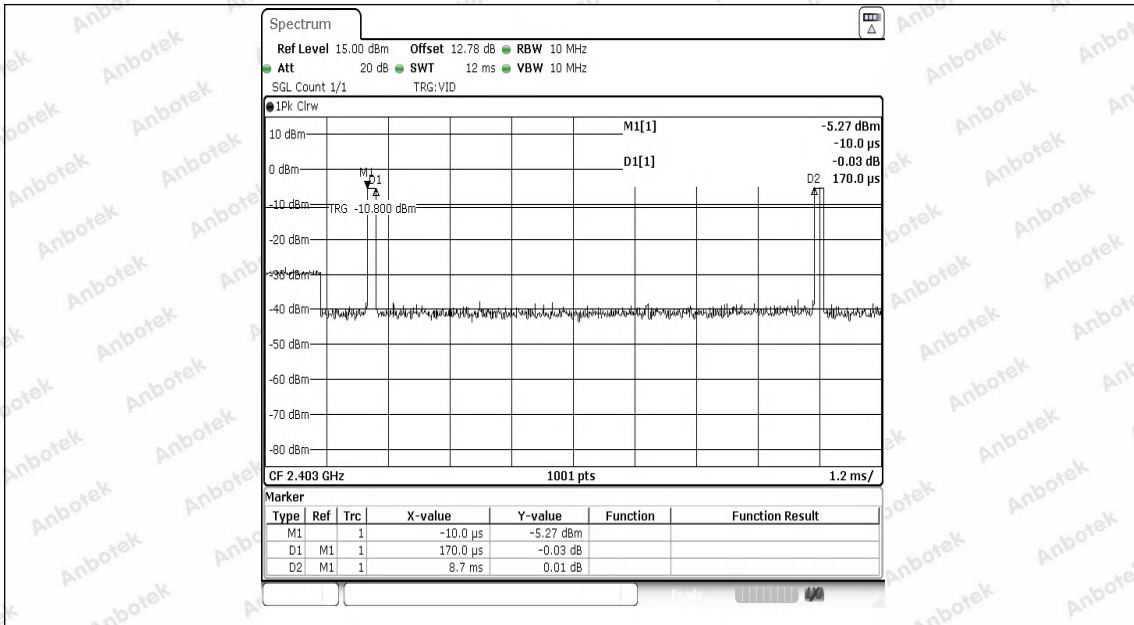
NTNV-2.4G-Ant1-2403
