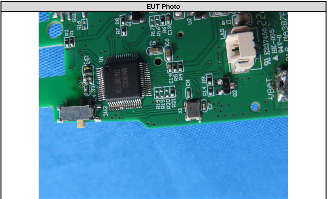
EUT Photo
